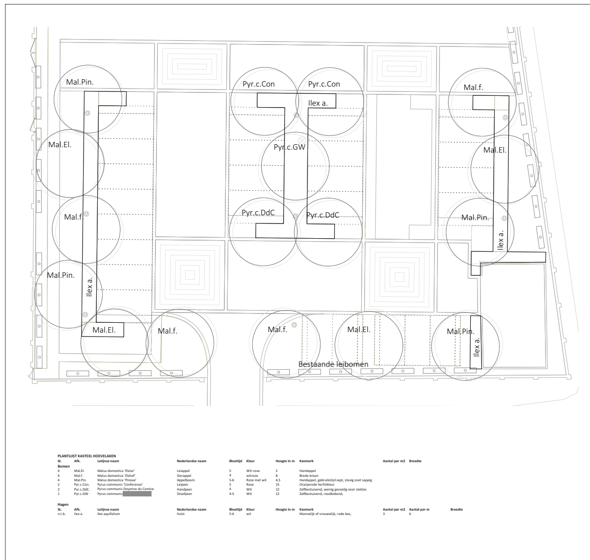
Beplantingsplan (D&V), aanleg najaar 2021.
