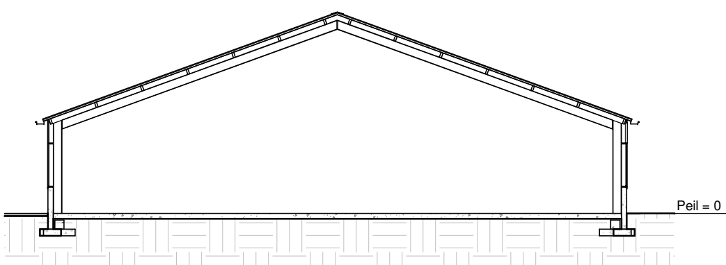
Doorsnede A-A 1: 200
