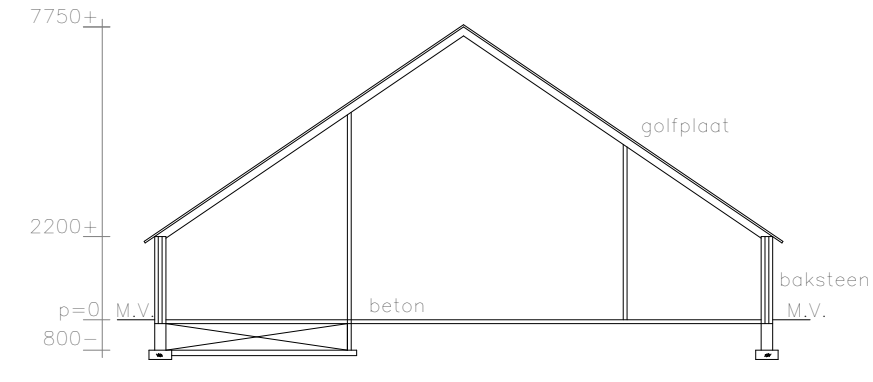
Doorsnede C-C 1: 200
