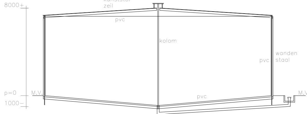
Doorsnede D-D 1: 200
