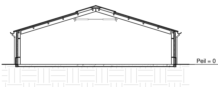
Doorsnede B-B 1: 200
