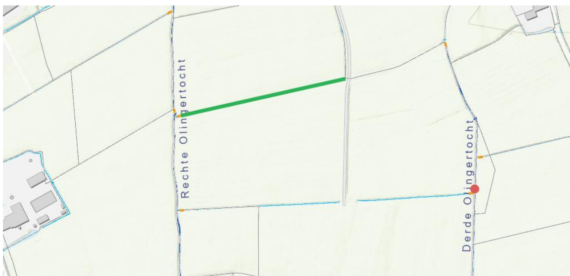
Figuur 1: Locatie van de activiteiten. De rode stip geeft globaal de locatie van de aan te leggen dam met duiker weer. De groene lijn geeft globaal de locatie weer waar het oppervlaktewaterlichaam gedeeltelijk wordt vergroot.
