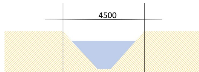
A. Dwarsprofiel van bestaande sloot (1: 100)
