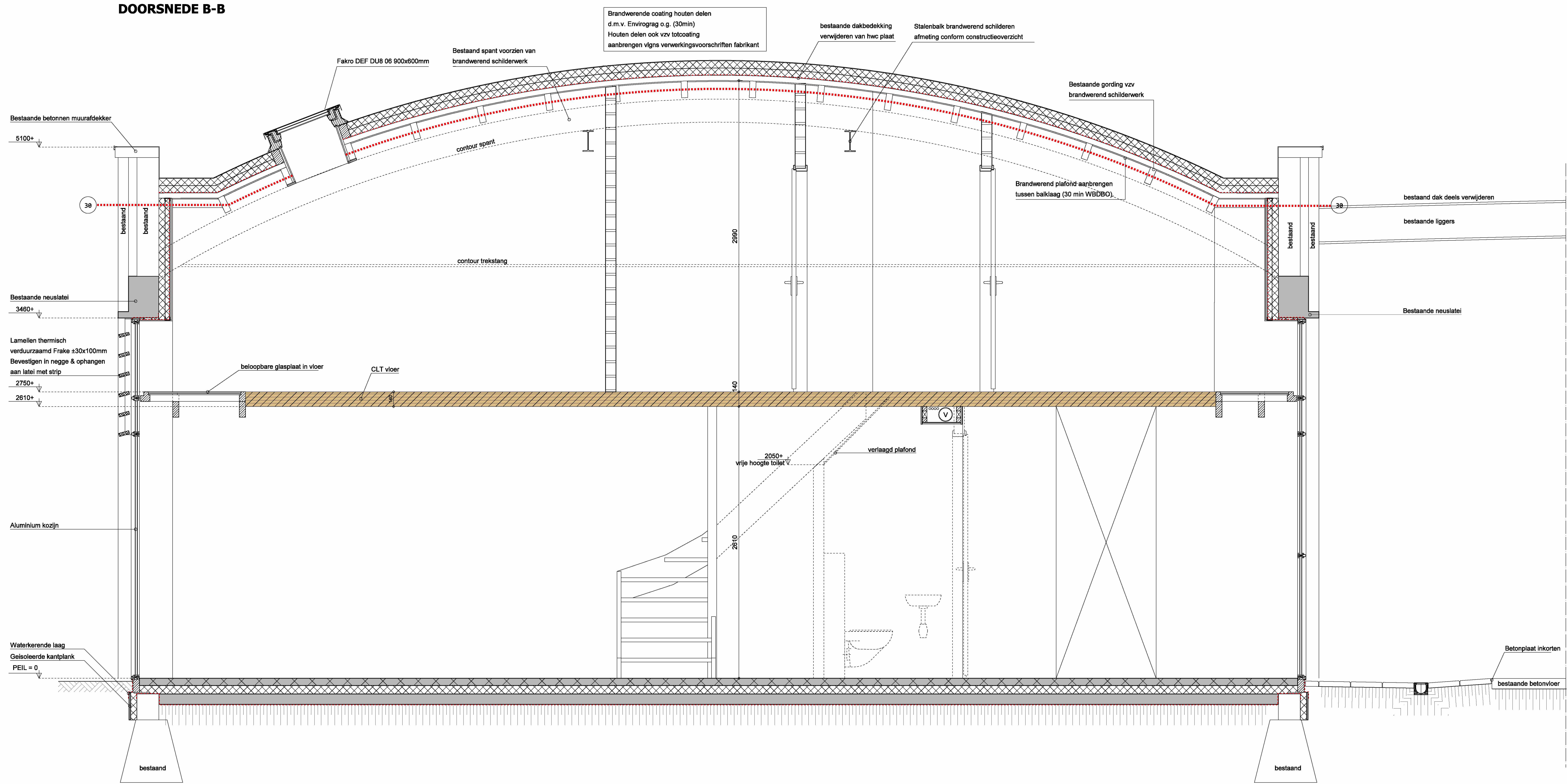
DOORSNEDE D-D
