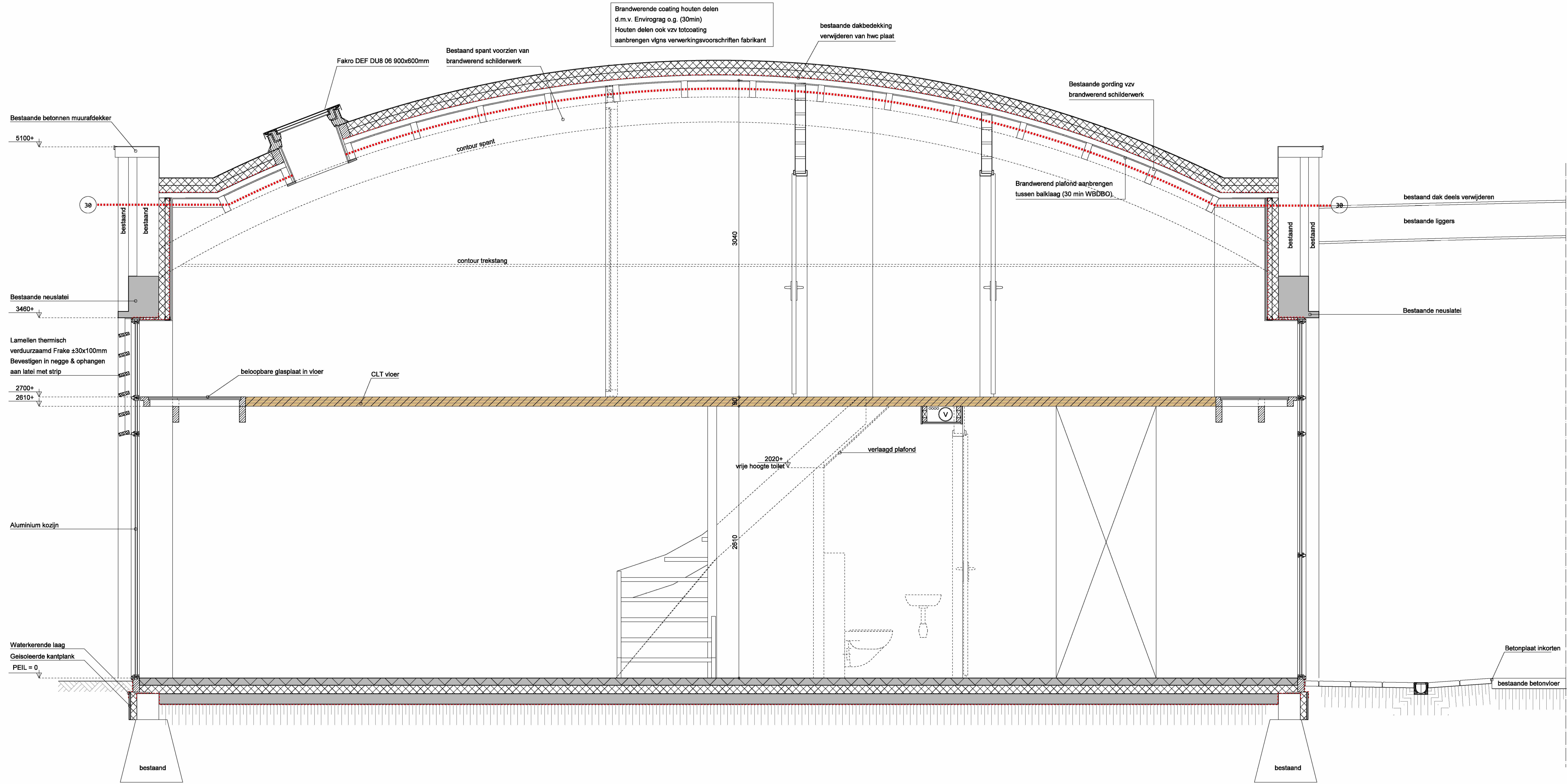
DOORSNEDE B-B
