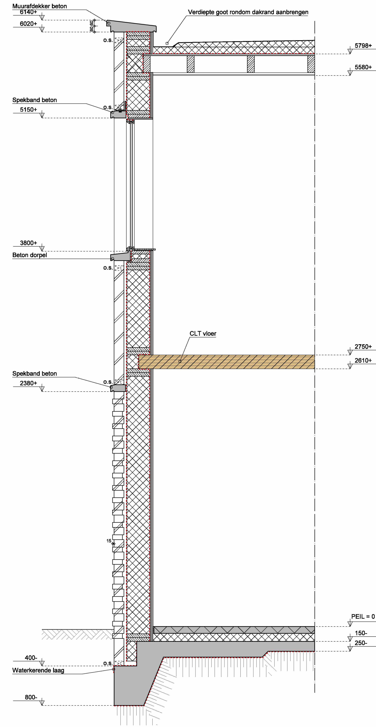
DOORSNEDE C
