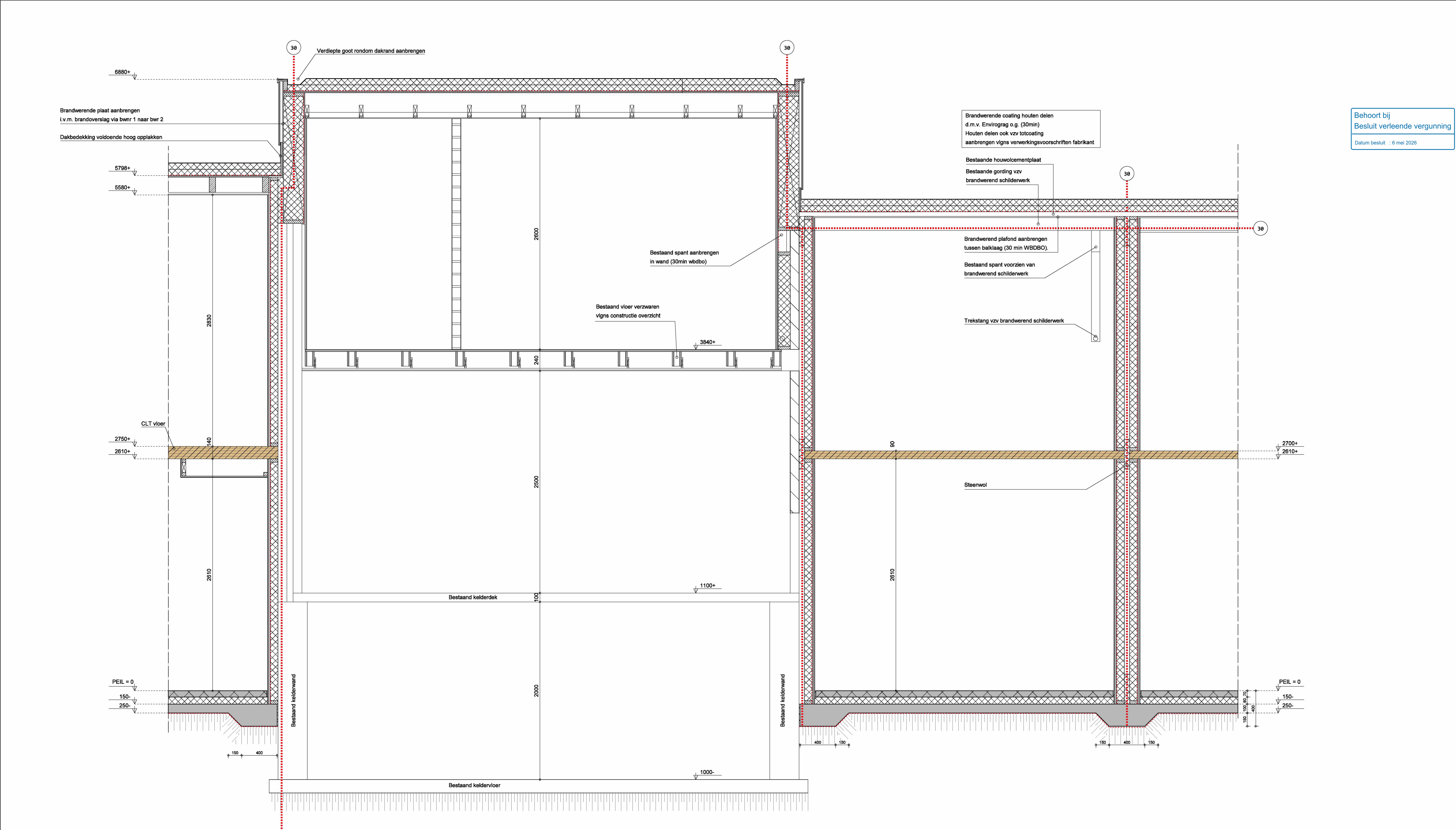
DOORSNEDE E-E
