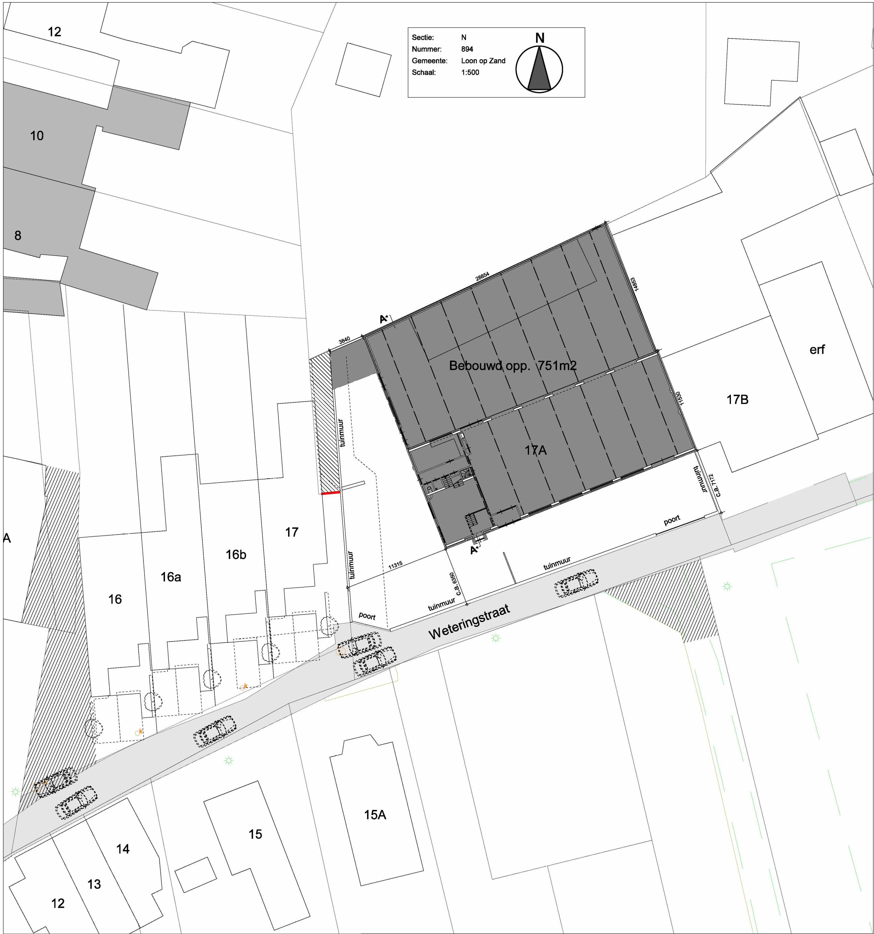
SITUATIE BESTAAND
