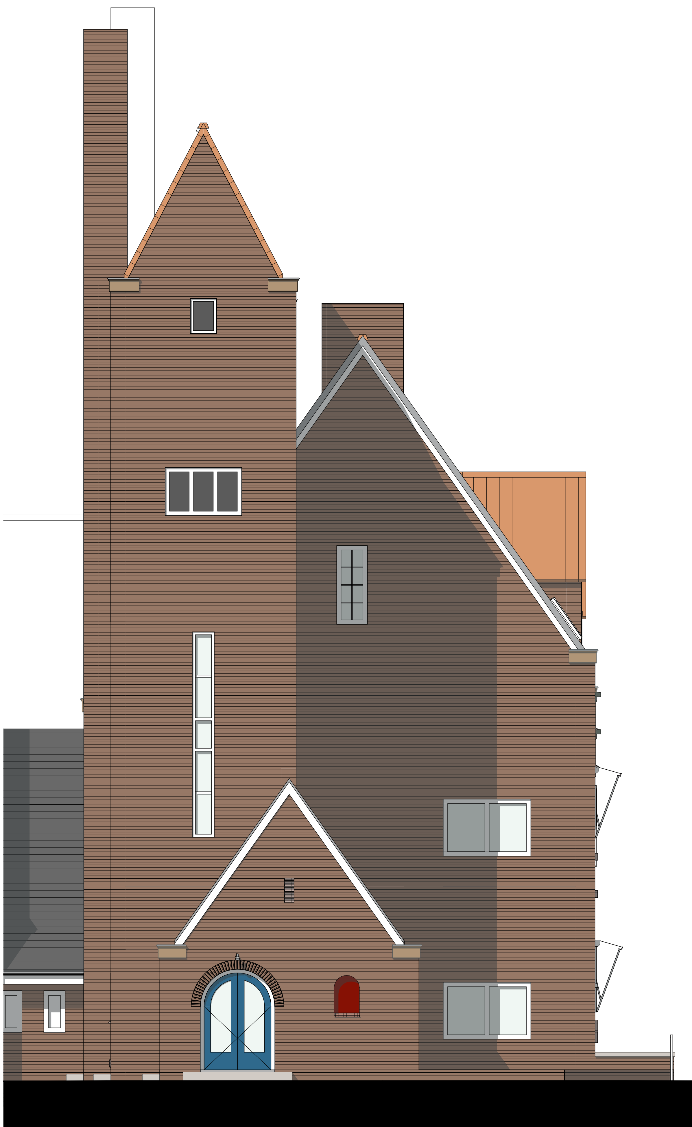
Noordwestgevel bouwdeel A (bestaand) - 1:50
