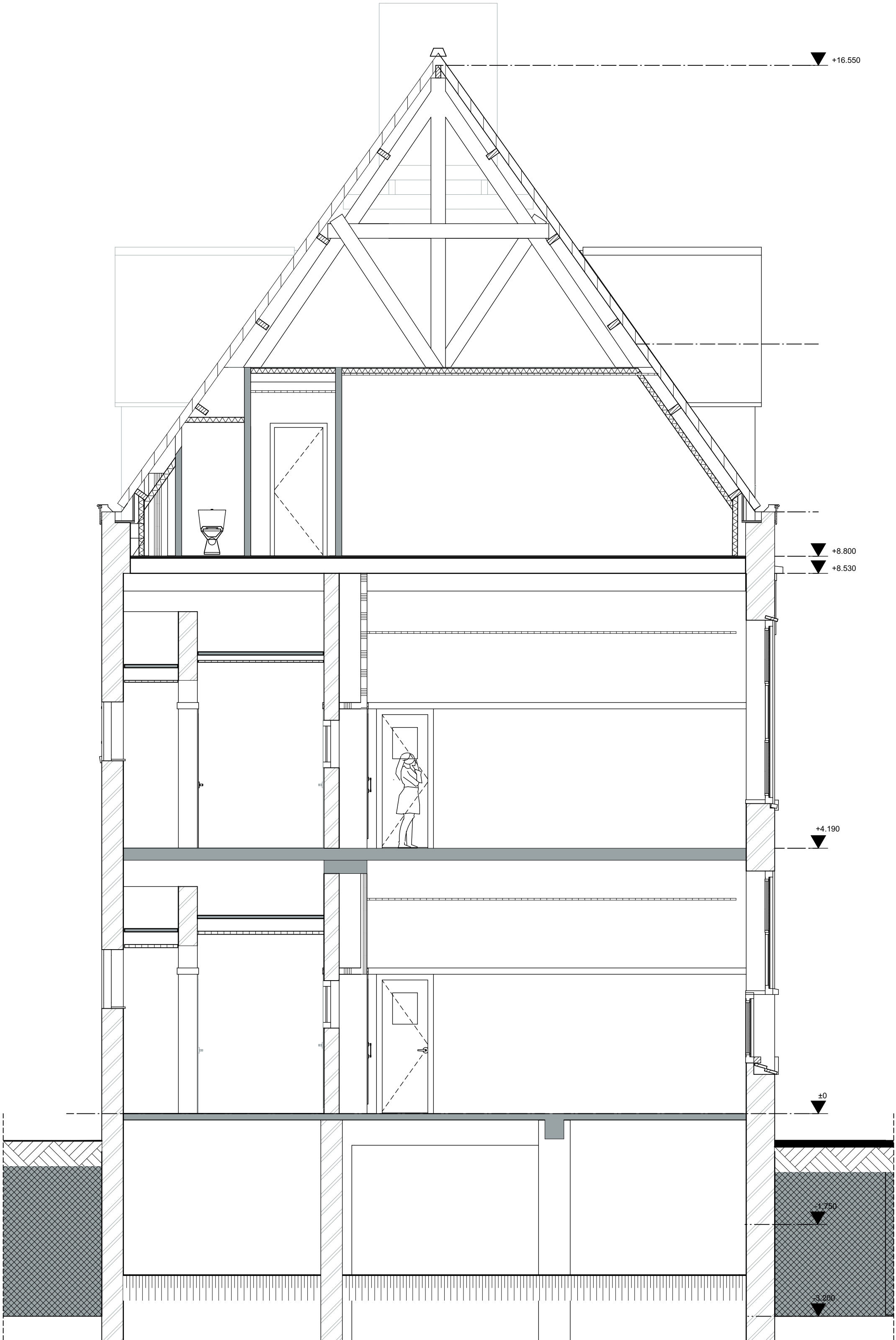
Doorsnede A1 - 1:50
