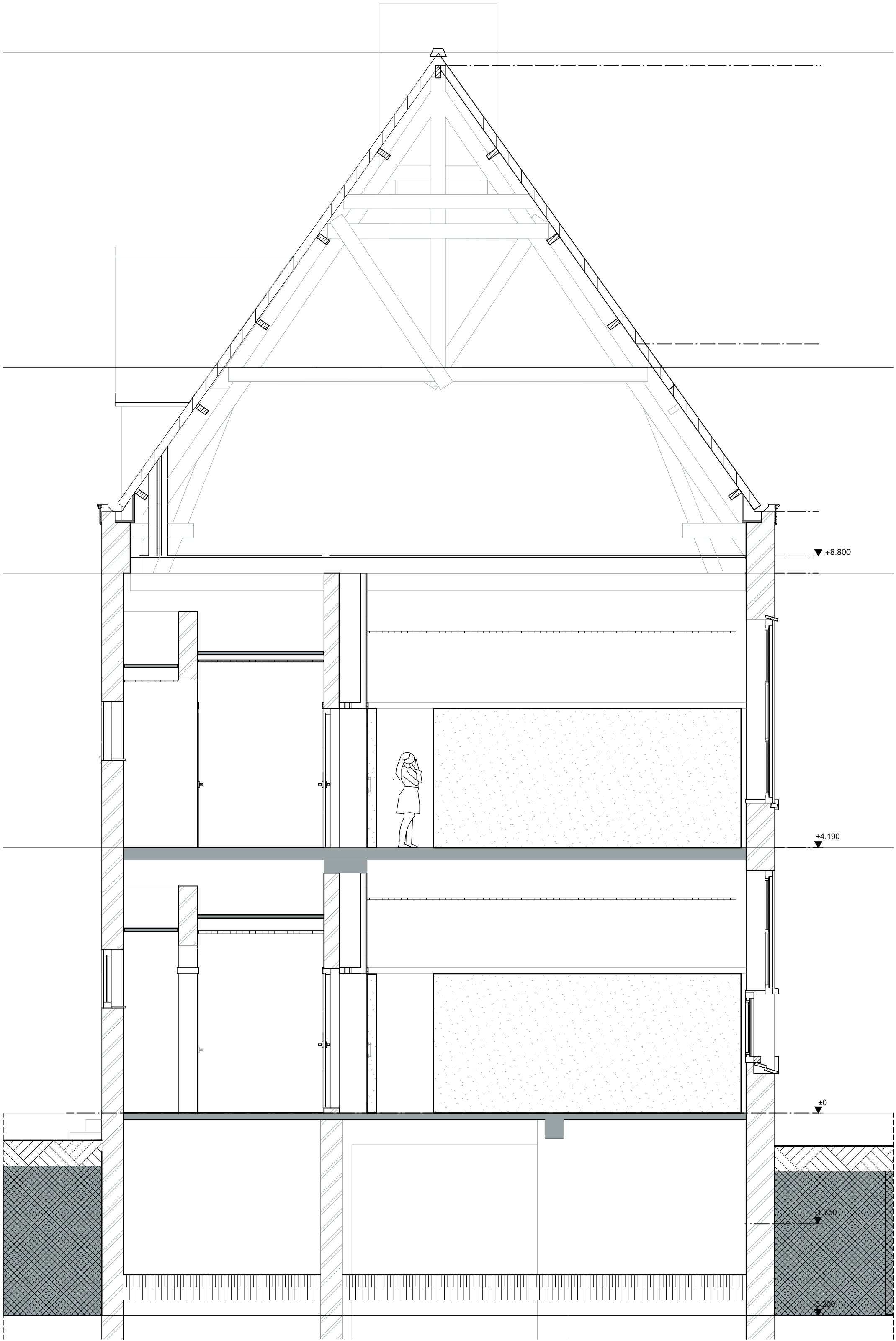
Doorsnede A2 - 1:50
