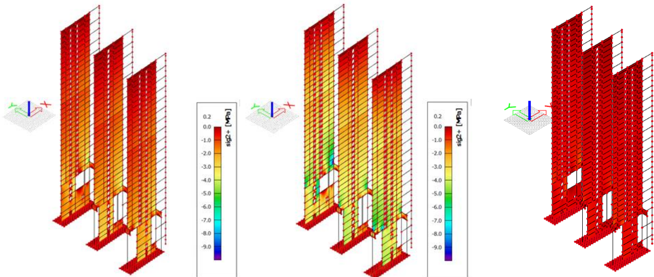
Figuur 10: Spanningen eigen gewicht (li), permanente belasting (mi), veranderlijke belasting (re)
