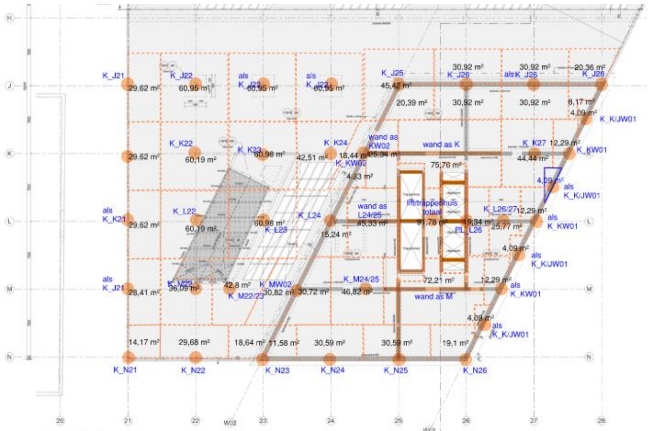
Figuur 3: Overzicht nummering berekende kolommen en wanden
