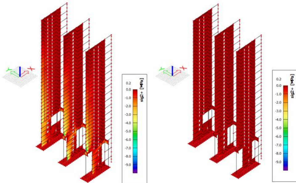
Figuur 11: Spanningen wind (li), geometrische imperfectie (re)
