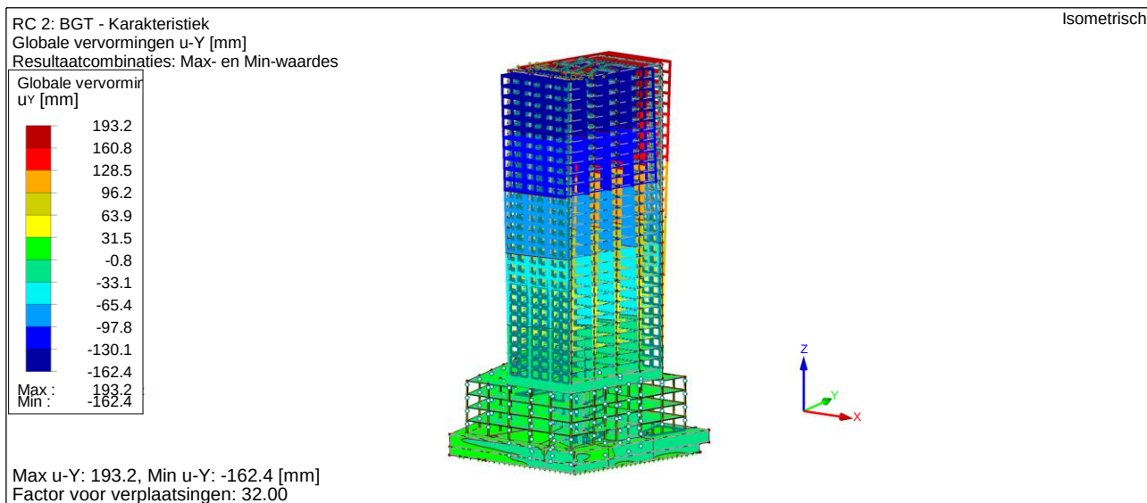
Figuur 9: Verplaatsingen aan de top volgens 3D rekenmodel (BGT)
