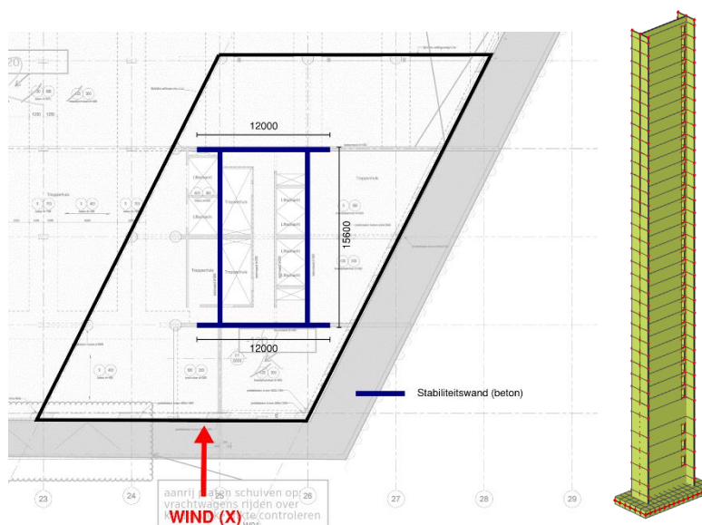
Figuur 7: (links) Stabiliteitsprincipe in lengterichting (Y-richting) over de volledige hoogte van het gebouw (rechts). 3D model van de stabiliteitswand in SCIA Engineer
