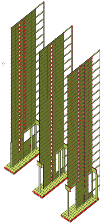
Figuur 6: 3D model van de stabiliteitswanden + outrigger constructie op de assen K, L, M
