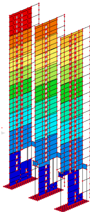
Figuur 8: Horizontale verplaatsingen aan de top (stabiliteit in dwarsrichting)
