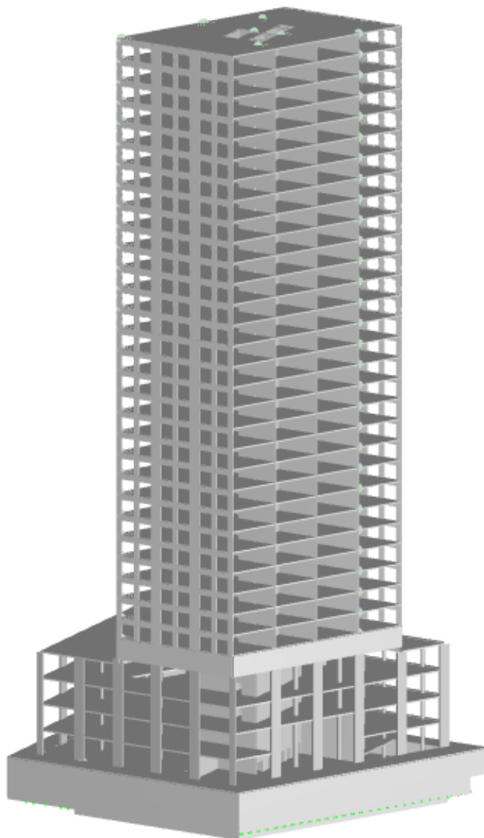
Figuur 1: Overzicht 3D-model EEM-berekening
