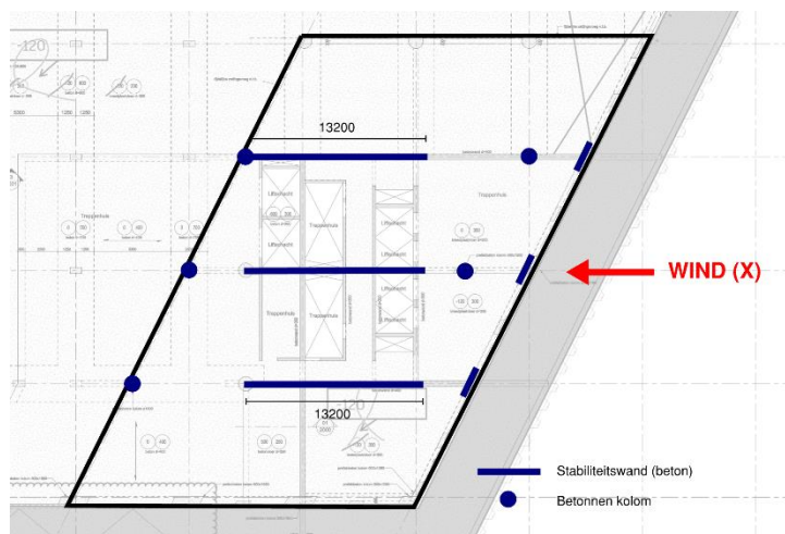
Figuur 5: Stabiliteitsprincipe van het outrigger-systeem in dwarsrichting (X-richting) voor de onderste verdiepingen
