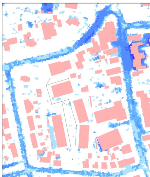
Afbeelding 3.4: Resultaat hydraulische berekening bui10 ( T=10 )
