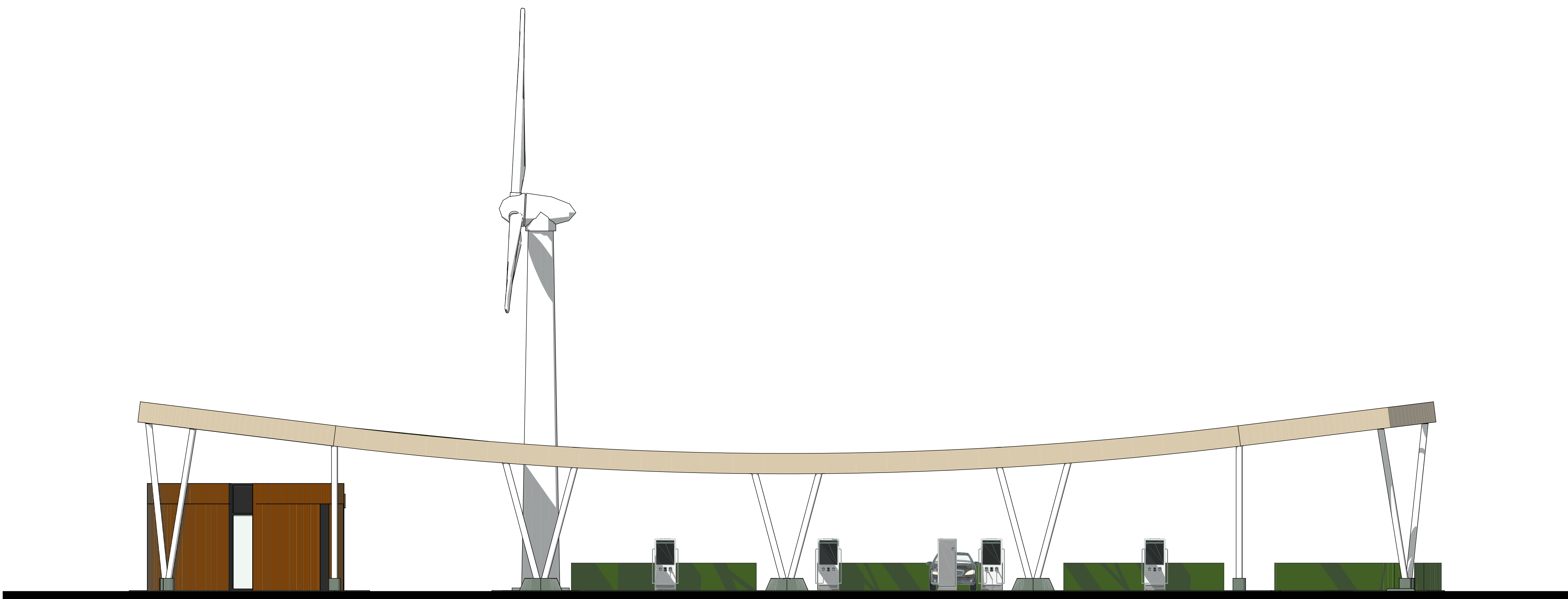
linkerzijgevel
