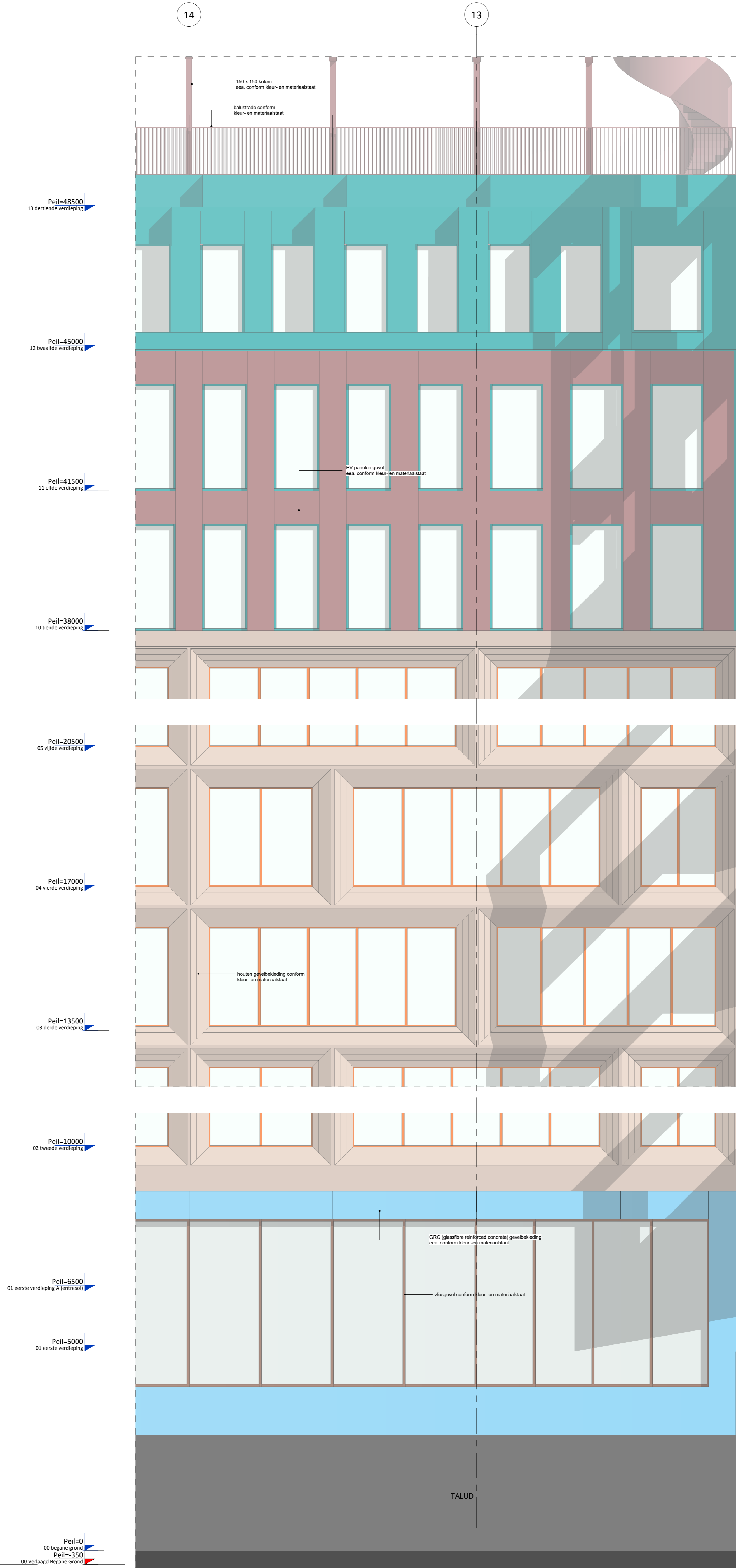
Gevel Noord - Blok C (01)
