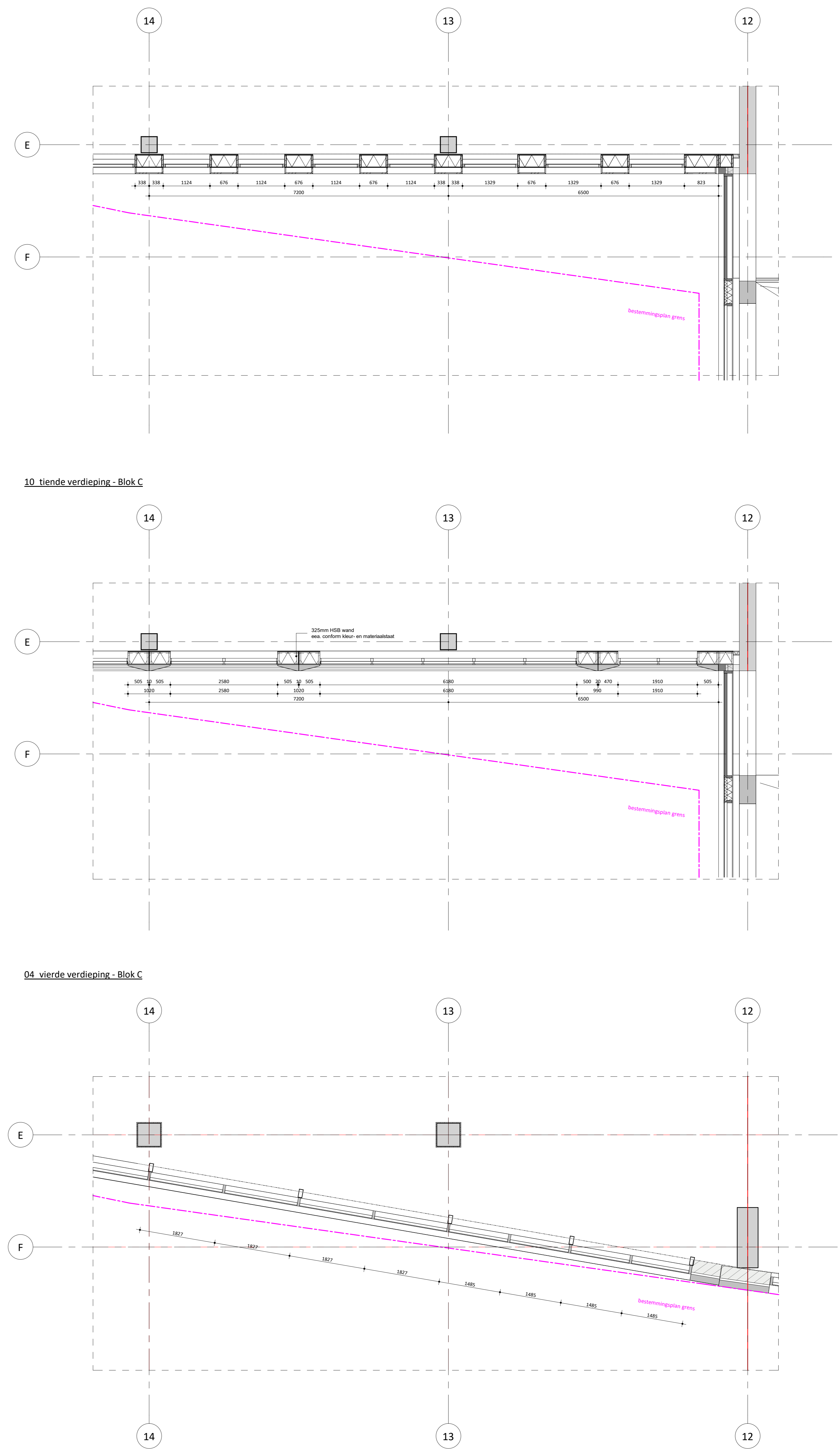
00e begane grond A (entresol) - Blok C
