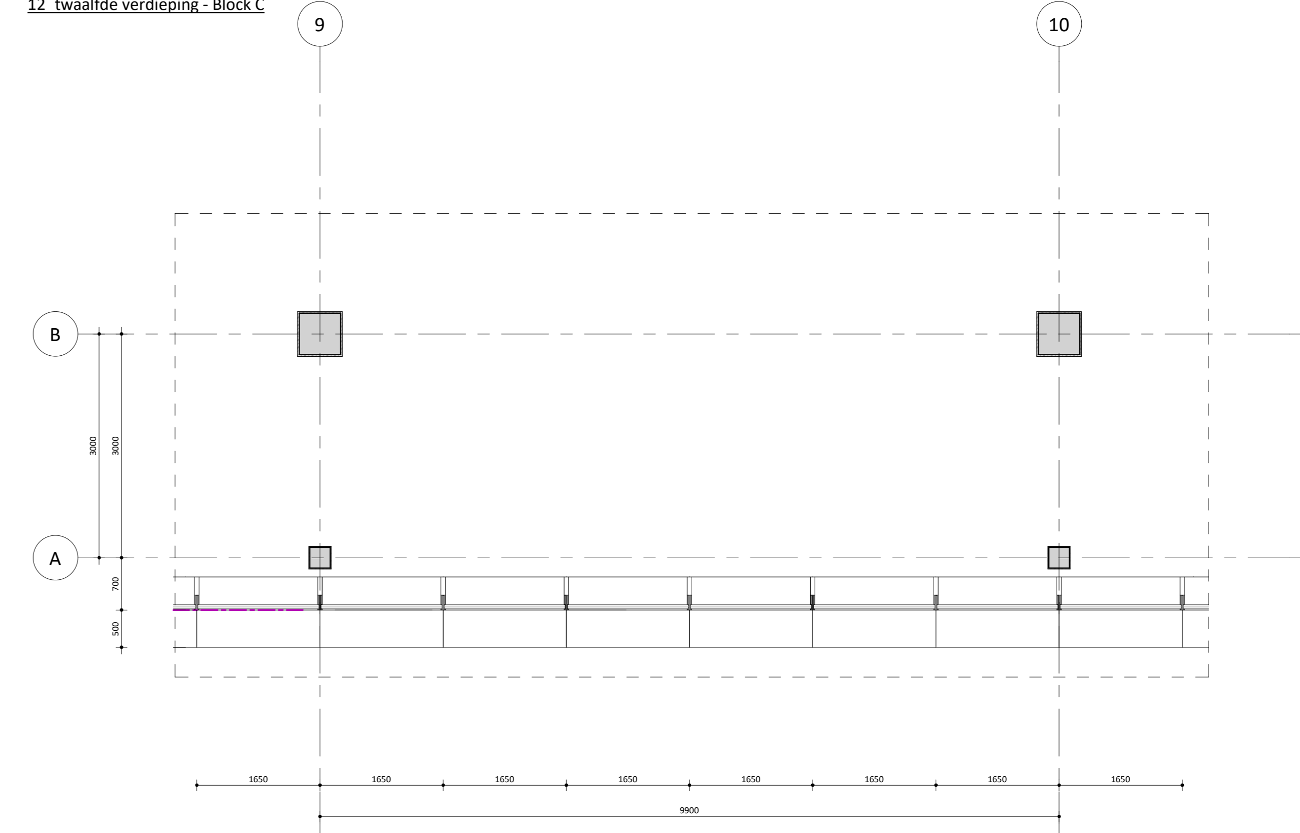
12 twaalfde verdieping - Blok C
