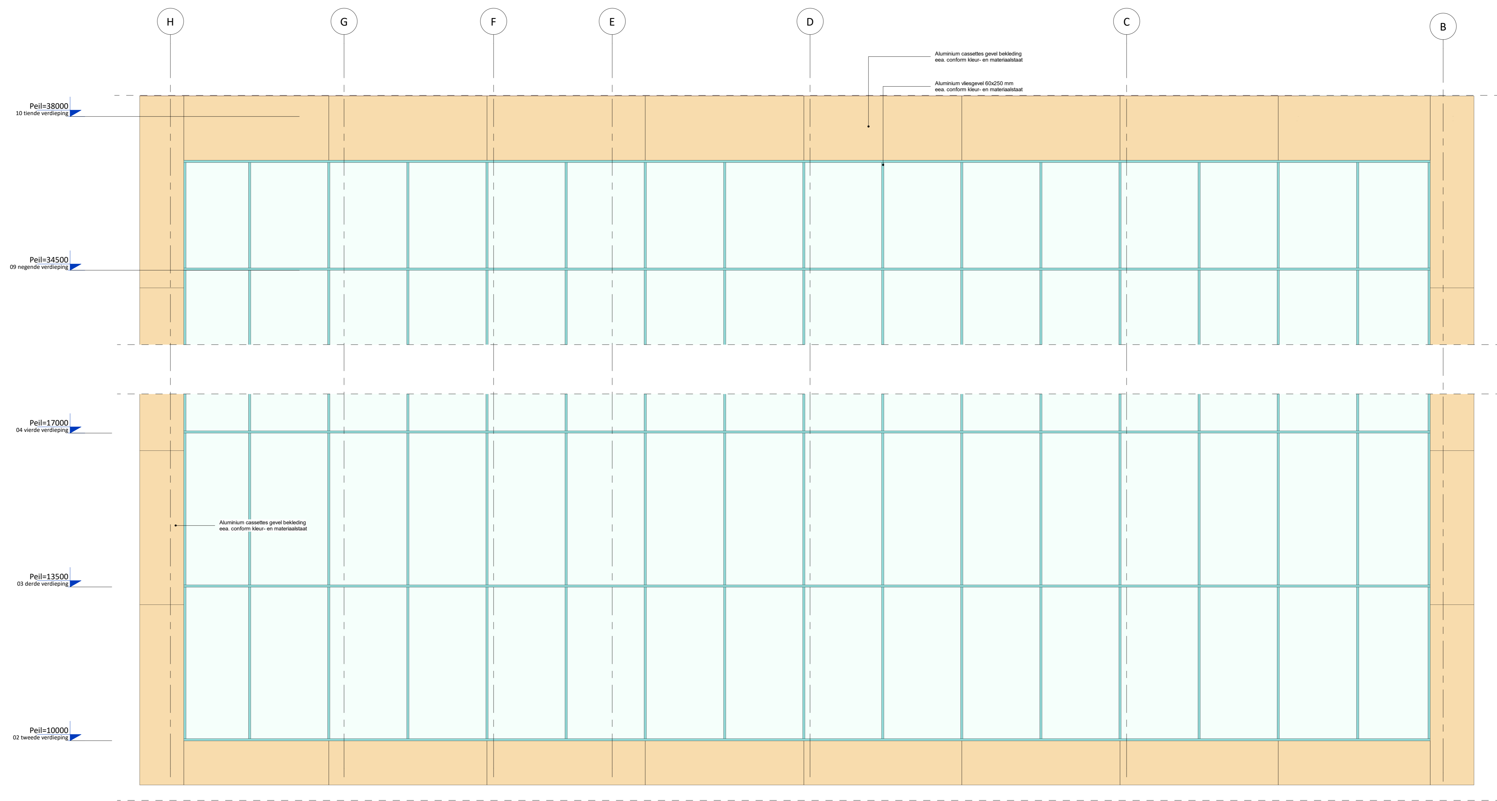
Gevel - Serre A (01)
