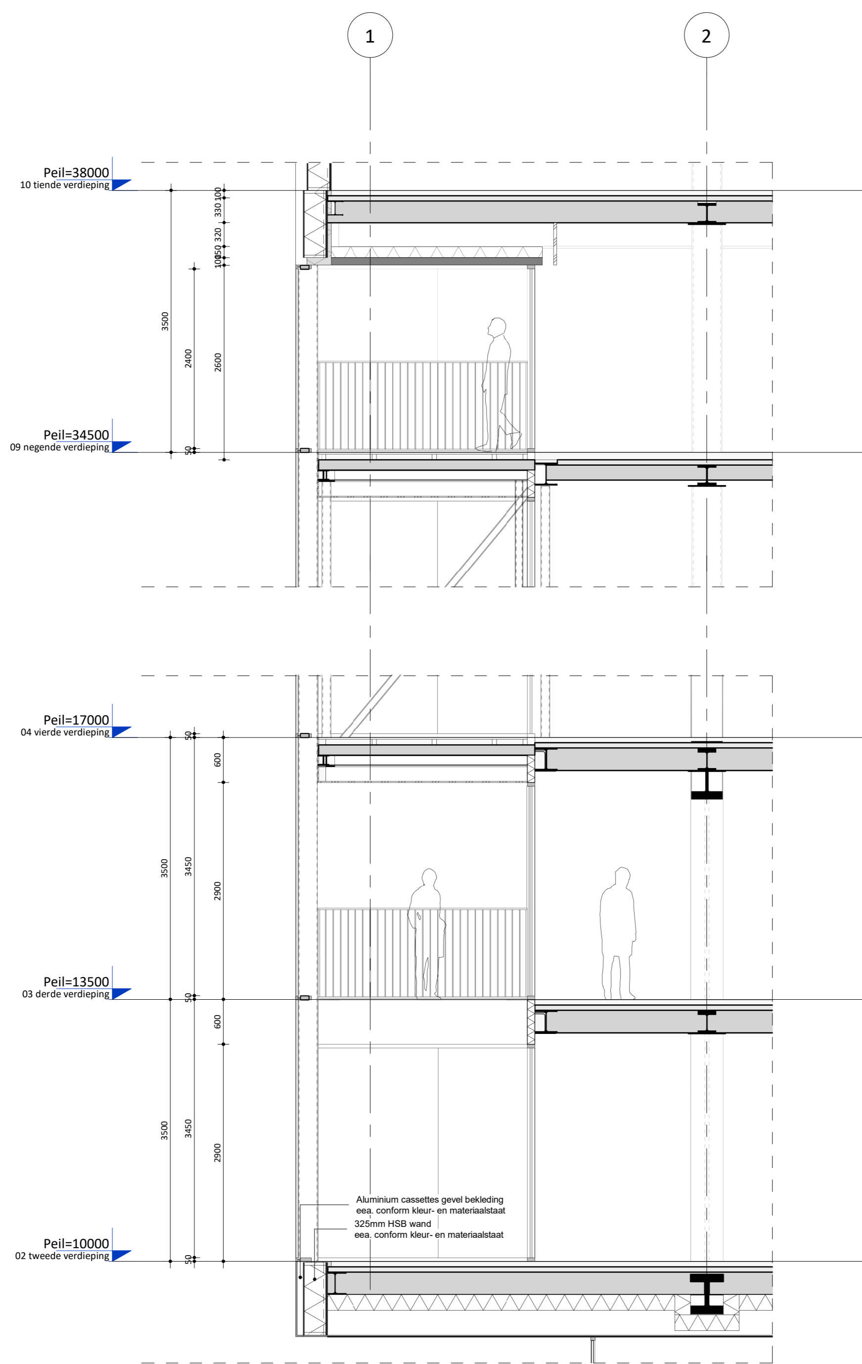
Doorsnede - Serre A (01)
