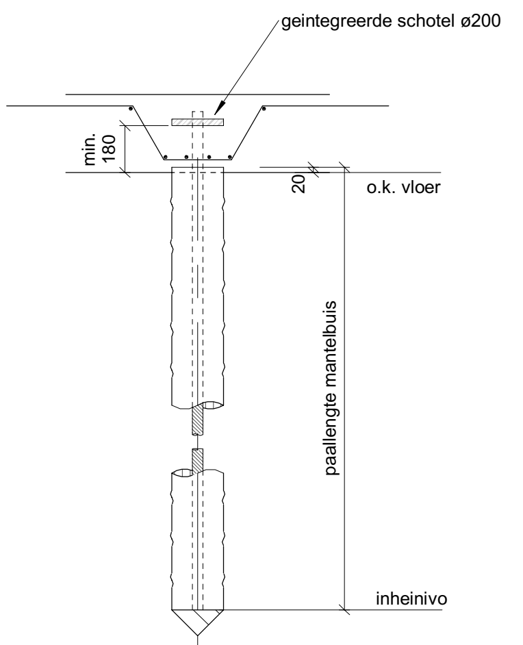
Alg. detail Gewi anker
