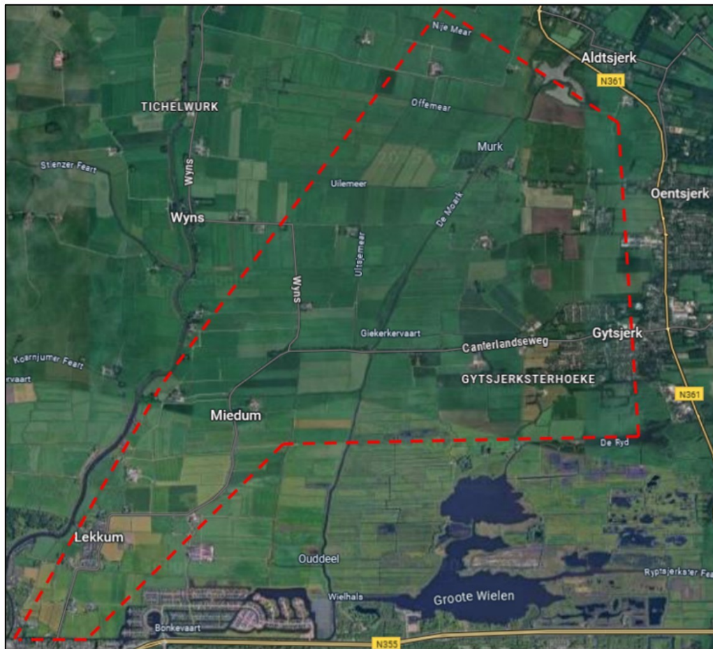
Overzicht plangebied Verbeteren waterhuishouding de Moark
