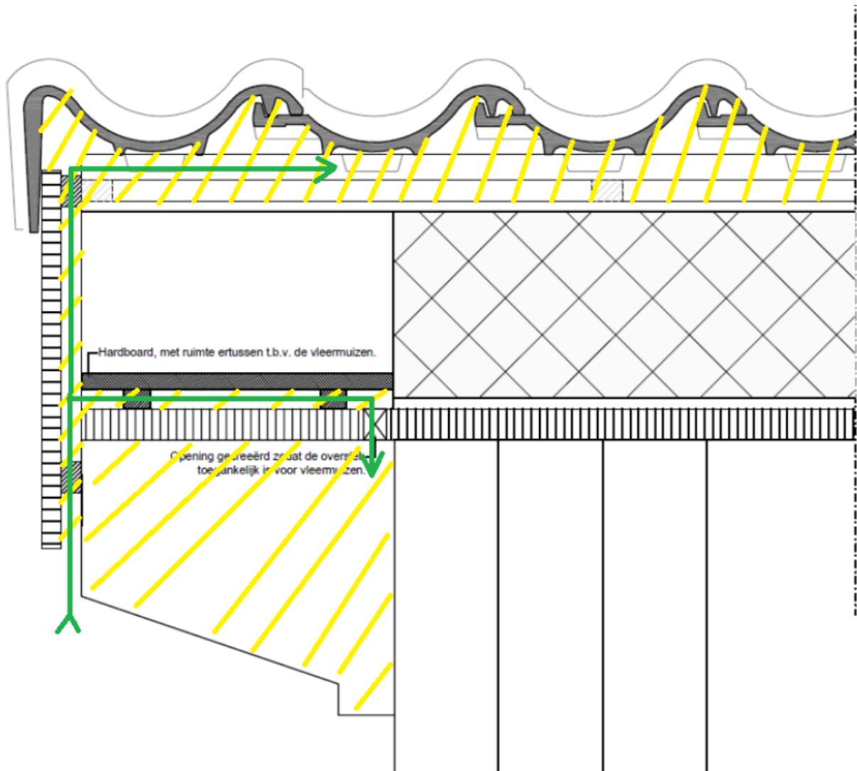
Figuur 1. Ruimten in de overstek en onder het dak toegankelijk voor vleermuizen (geel gearceerd) en de kruiproute (groene lijn).
