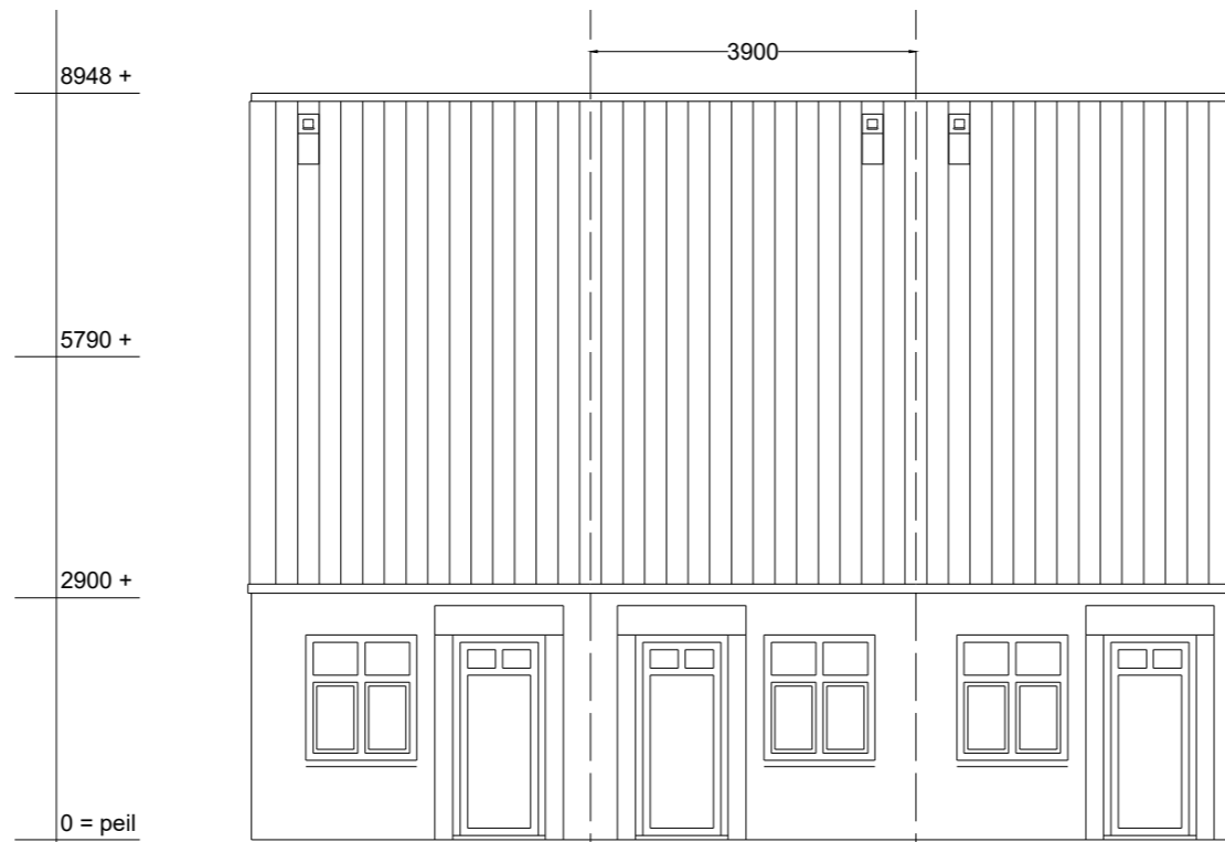
VOORGEVEL BESTAAND
