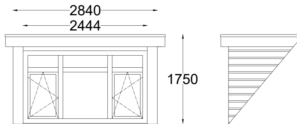
AANZICHT DAKKAPEL
