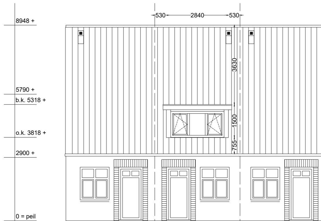
VOORGEVEL NIEUW
