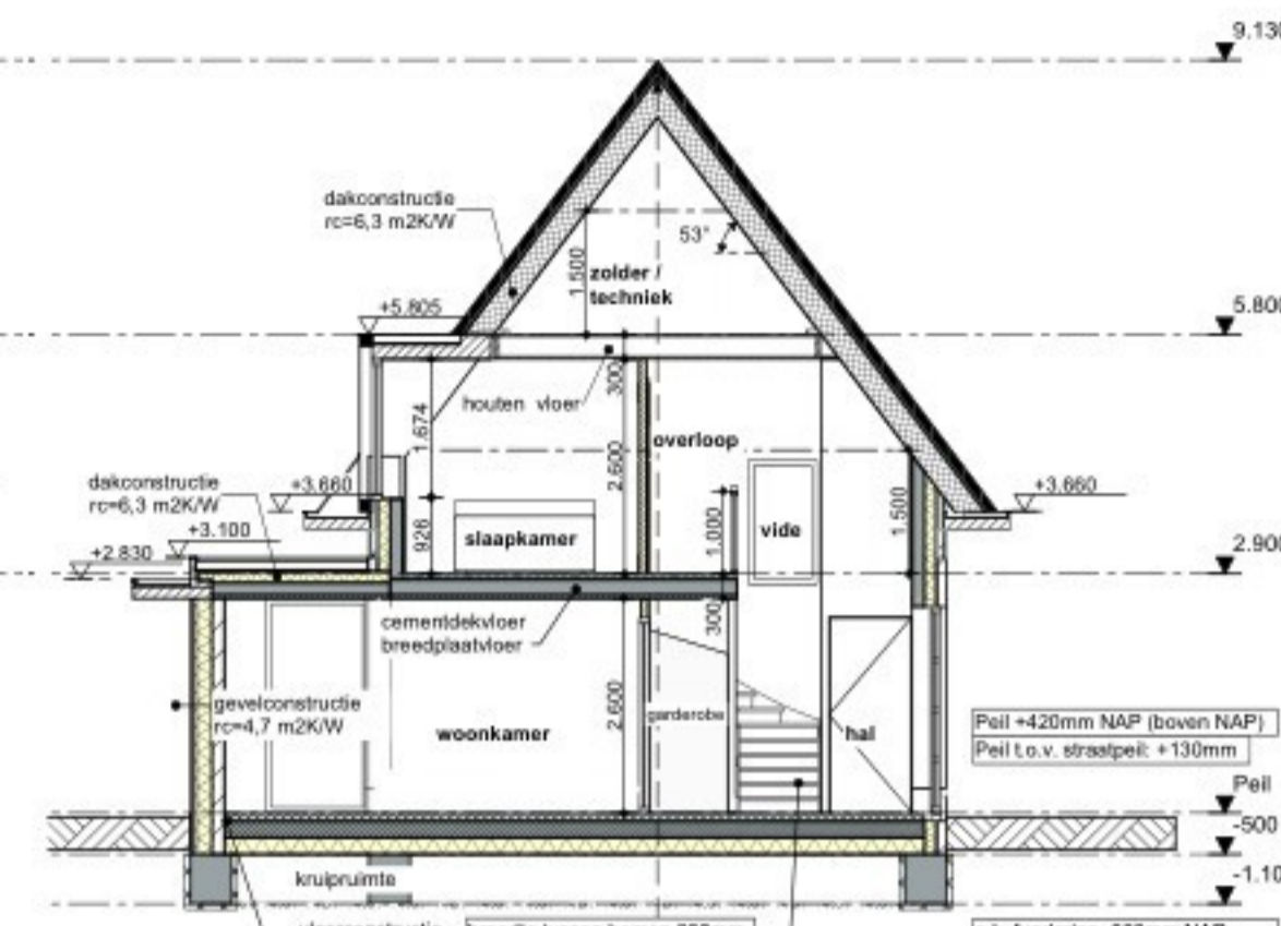
dwarsdoorsnede (D)
