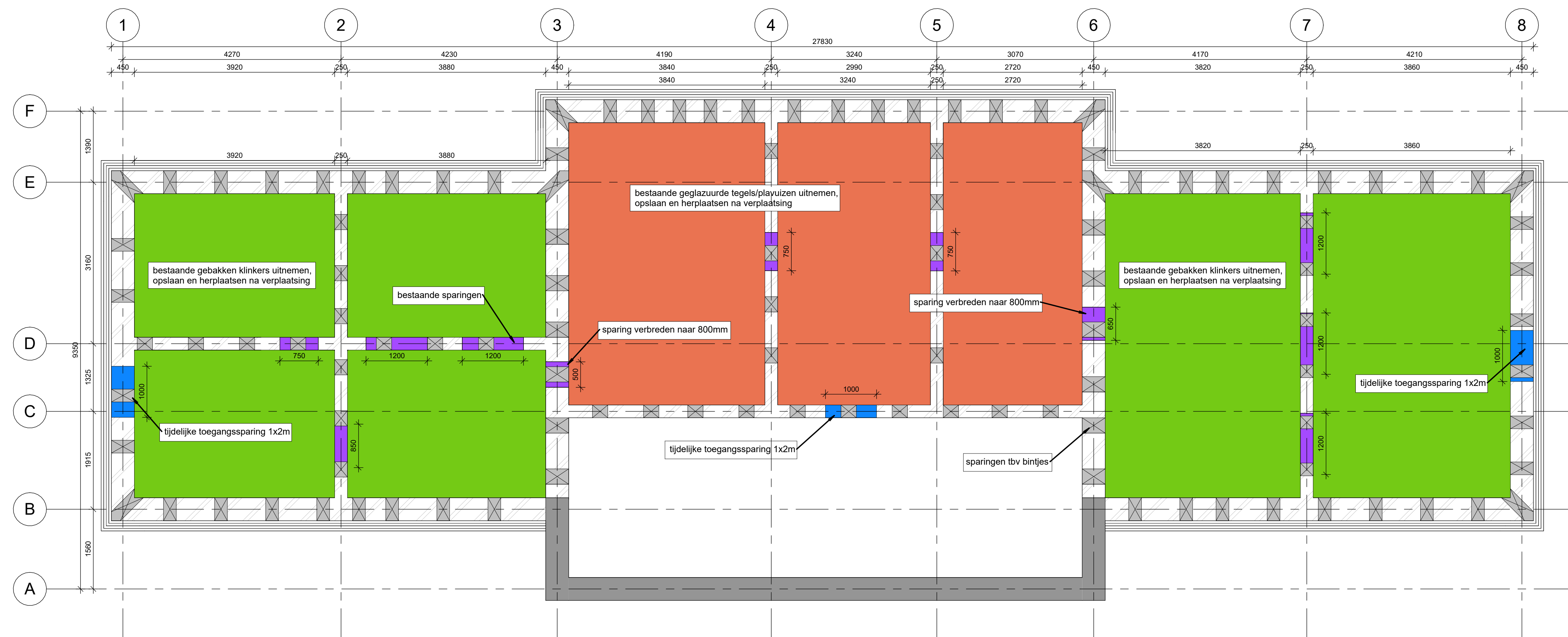
SLOOPWERKZAAMHEDEN IN KELDER 1 : 50
