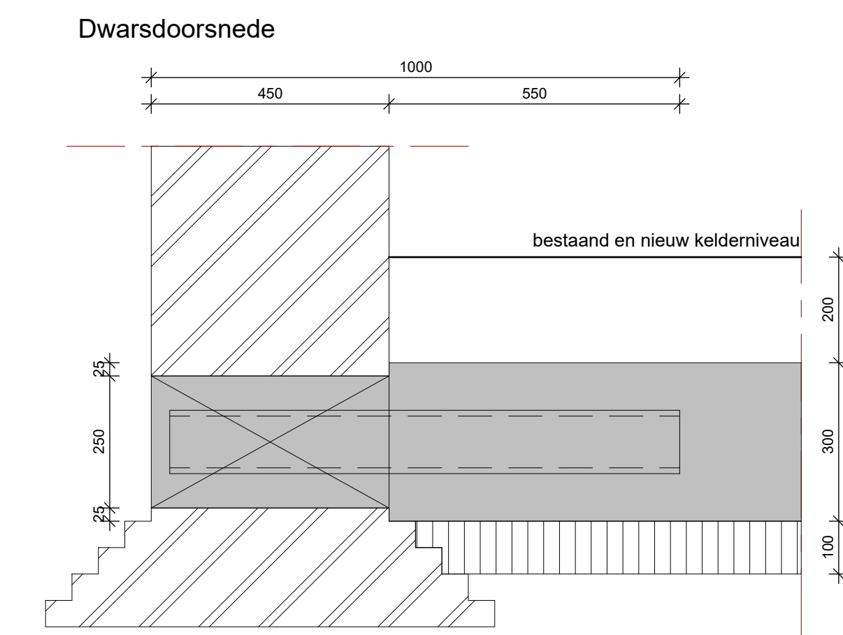
INKASSING BUITENWAND 1 : 10
