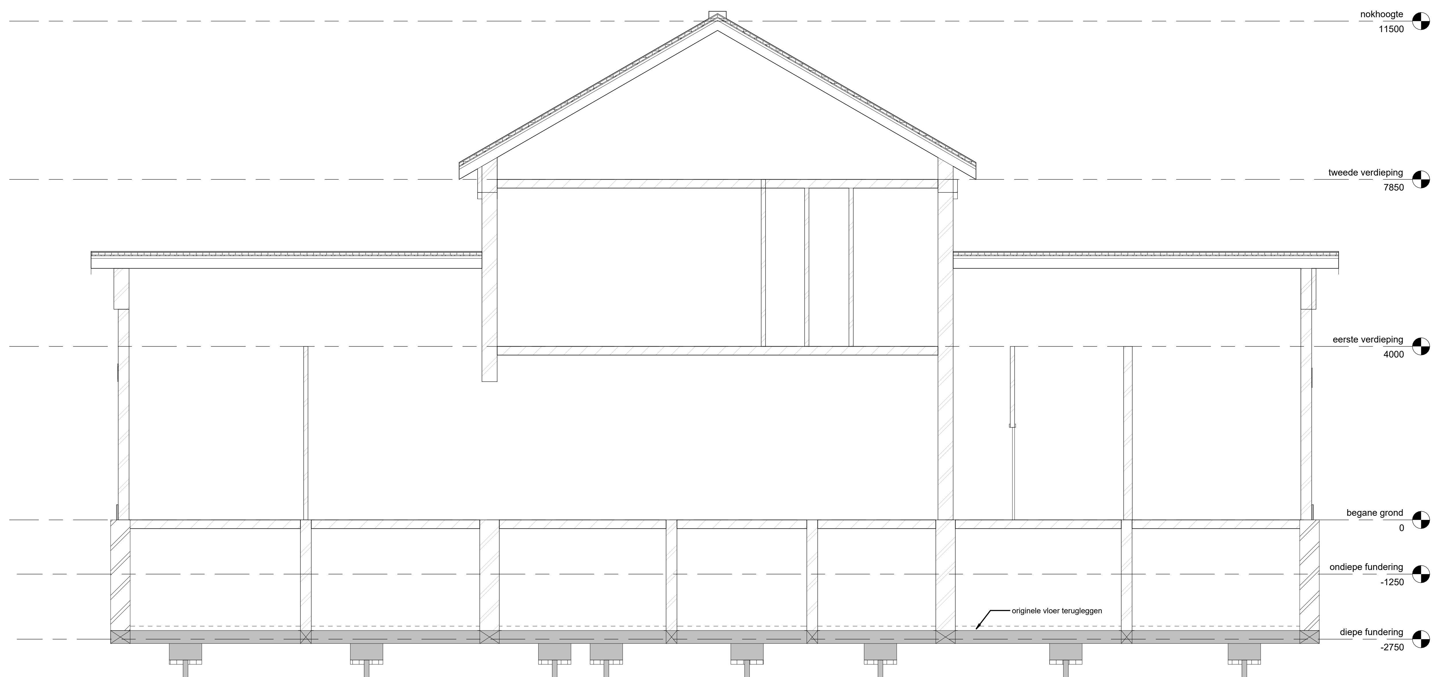
DOORSNEDE BB NIEUWE SITUATIE 1 : 50
