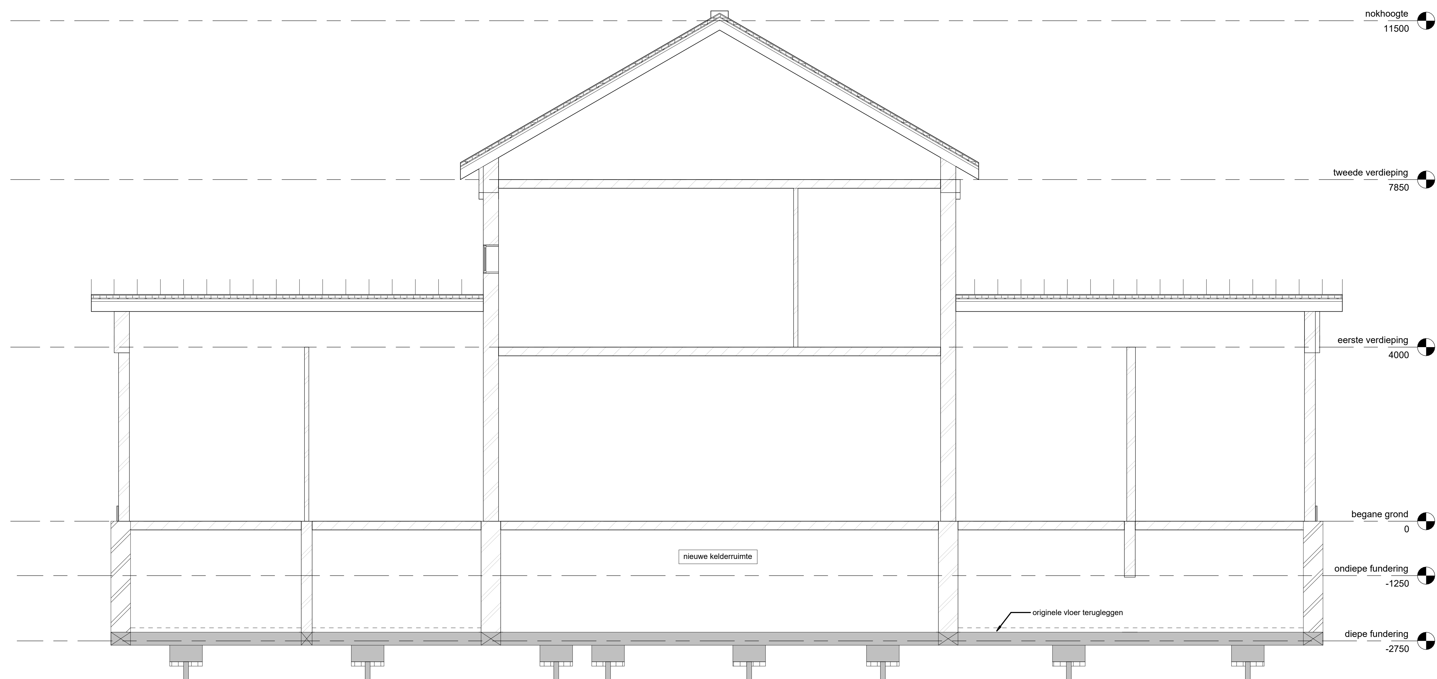
DOORSNEDE AA NIEUWE SITUATIE 1 : 50
