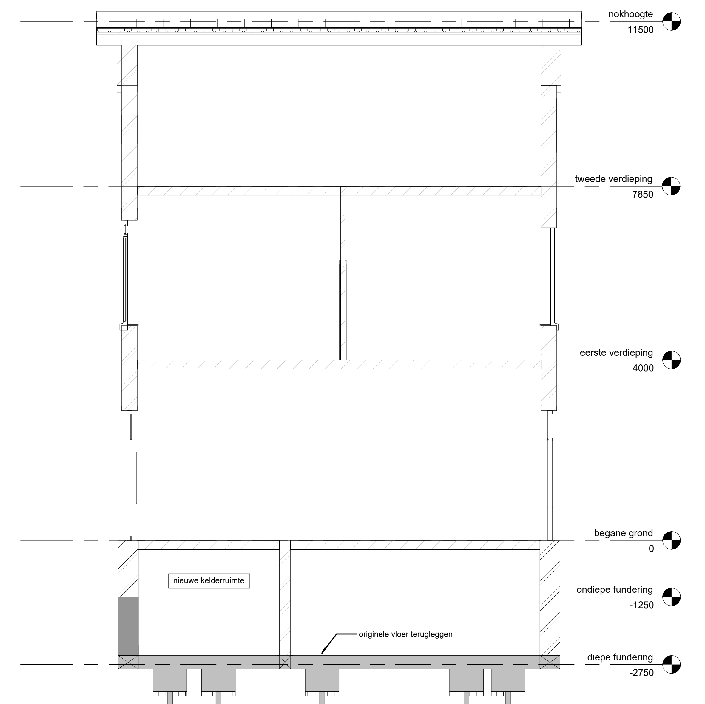
DOORSNEDE CC SITUATIE 1 : 50
