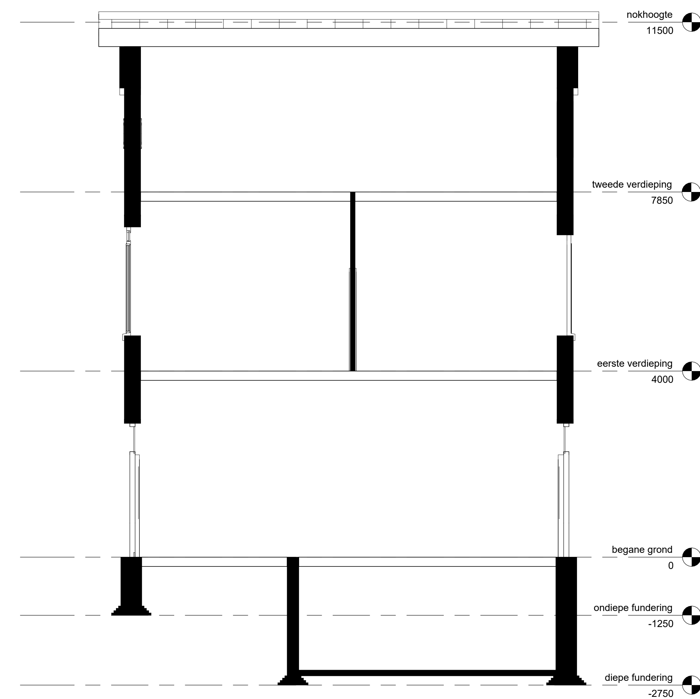
DOORSNEDE CC
