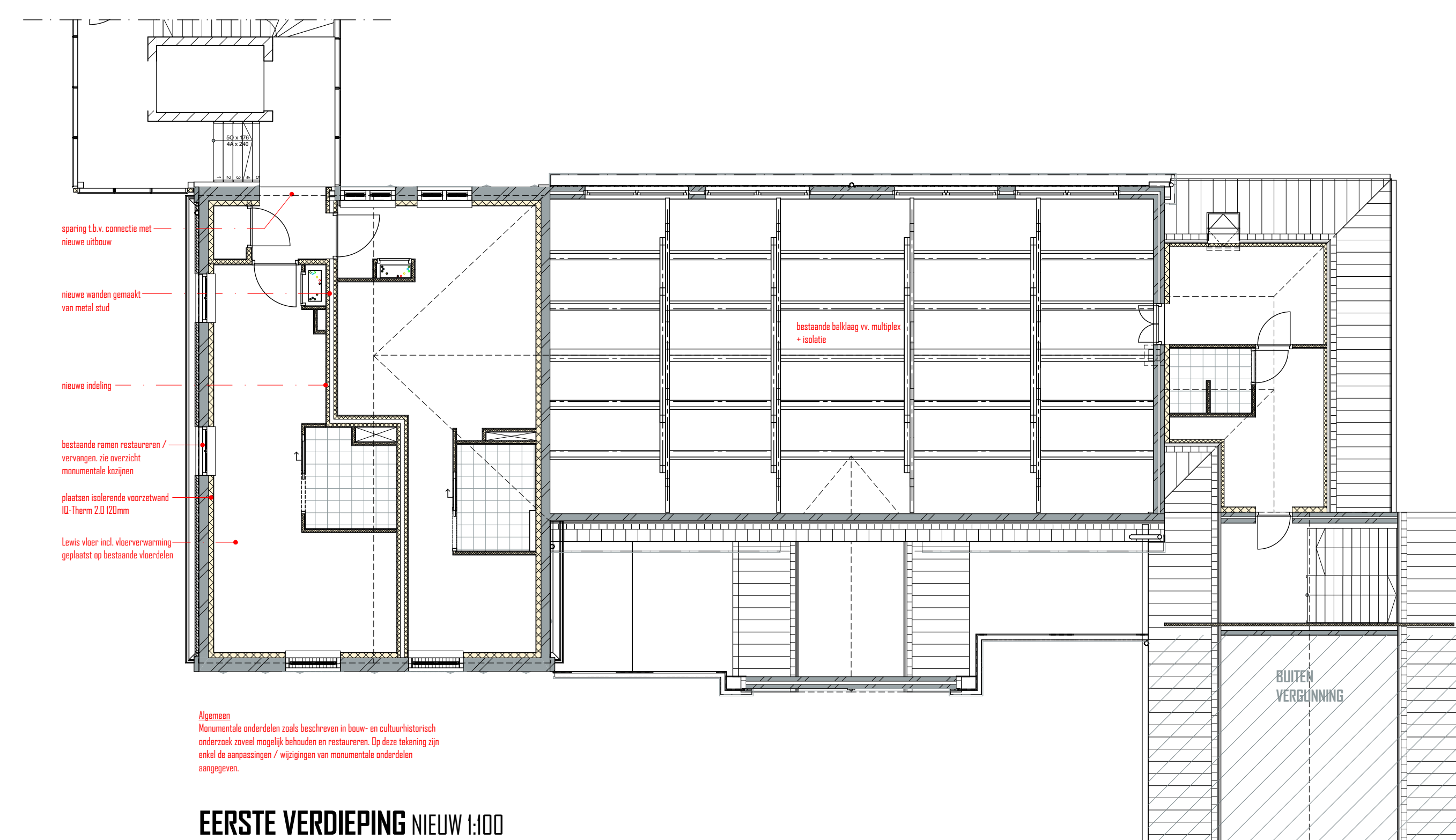
EERSTE VERDIEPING NIEUW I:100
