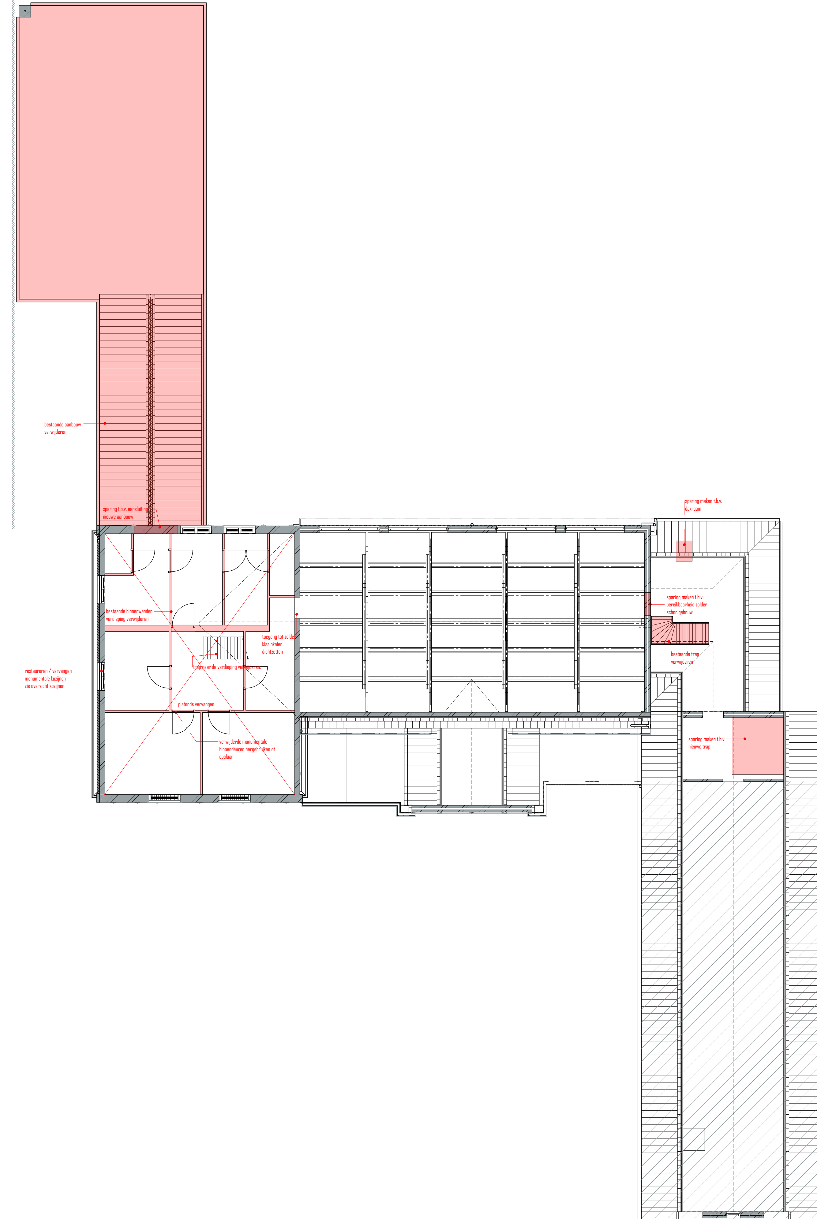
EERSTE VERDIEPING BESTAAND I:100
