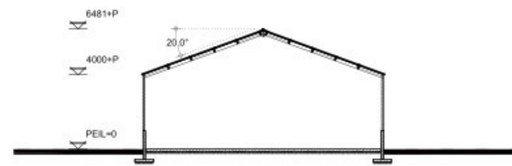
DOORSNEDE A-A GEBOUWR 1
