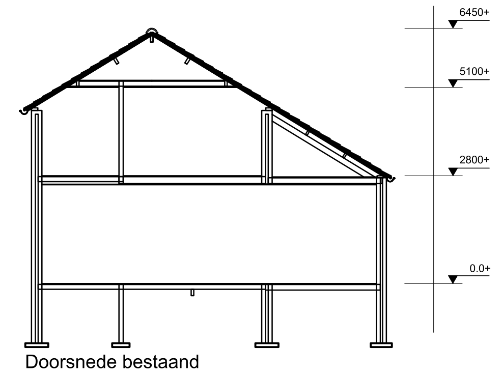
Doorsnede bestaand
