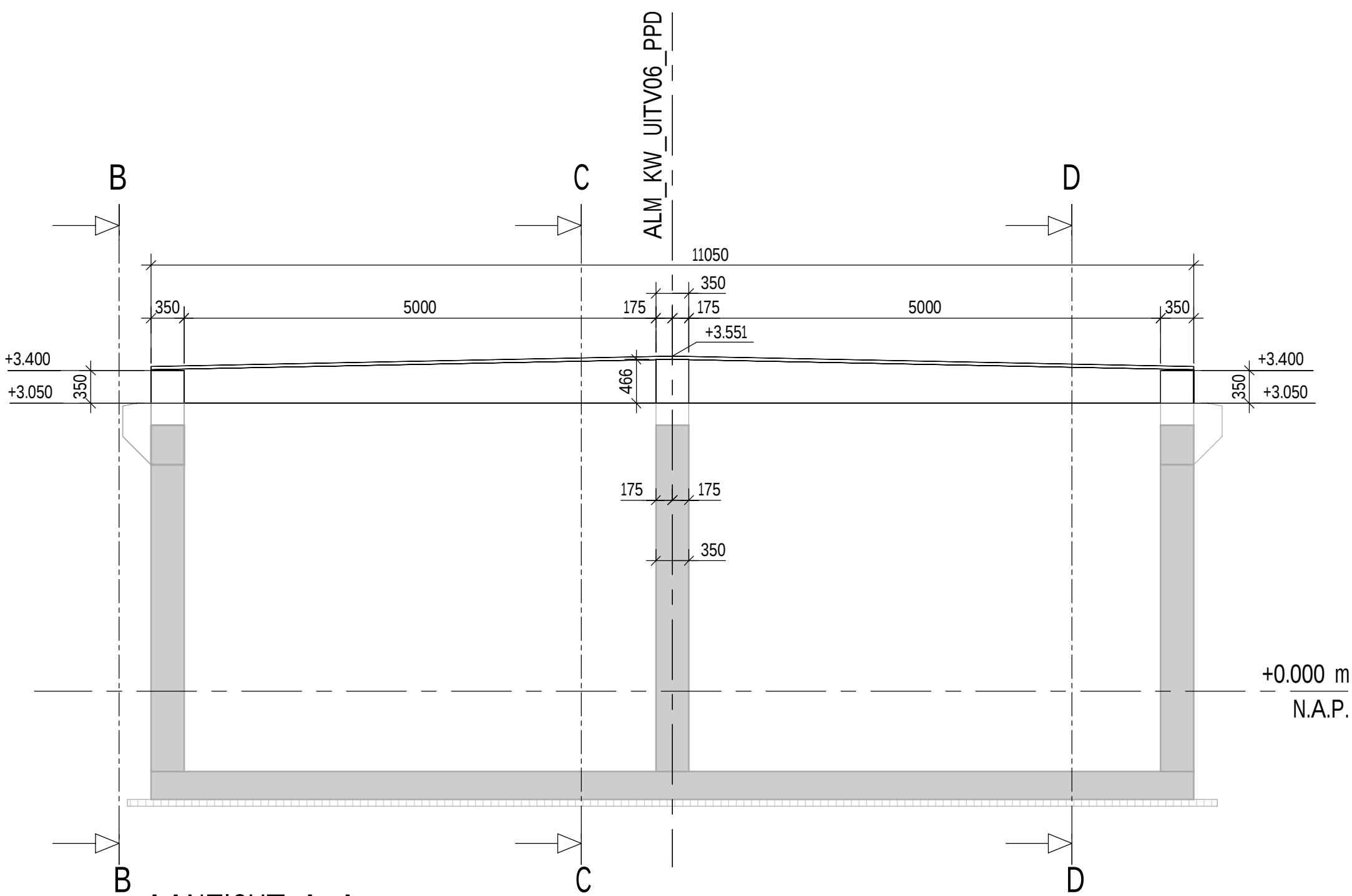
AANZICHT A-A schaal: 1 : 50
