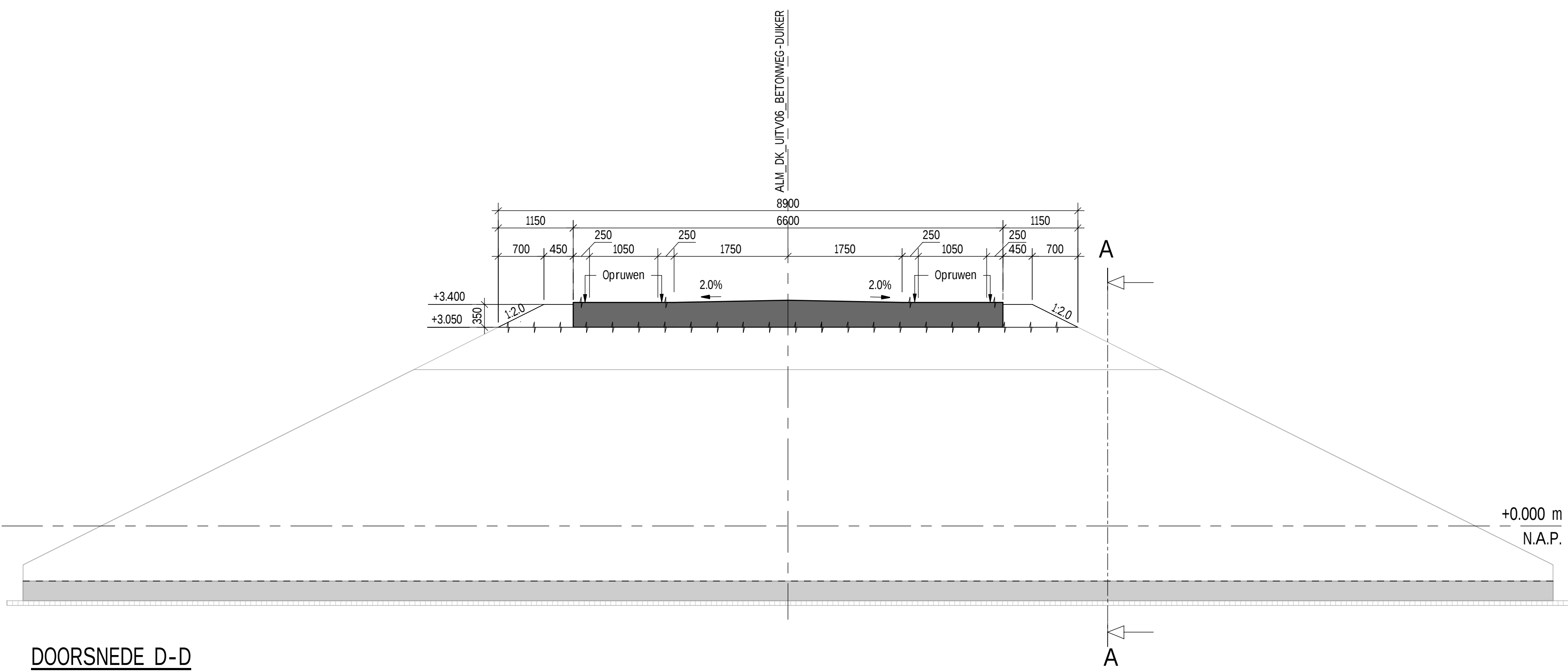
DOORSNEDE D-D schaal: 1 : 50
