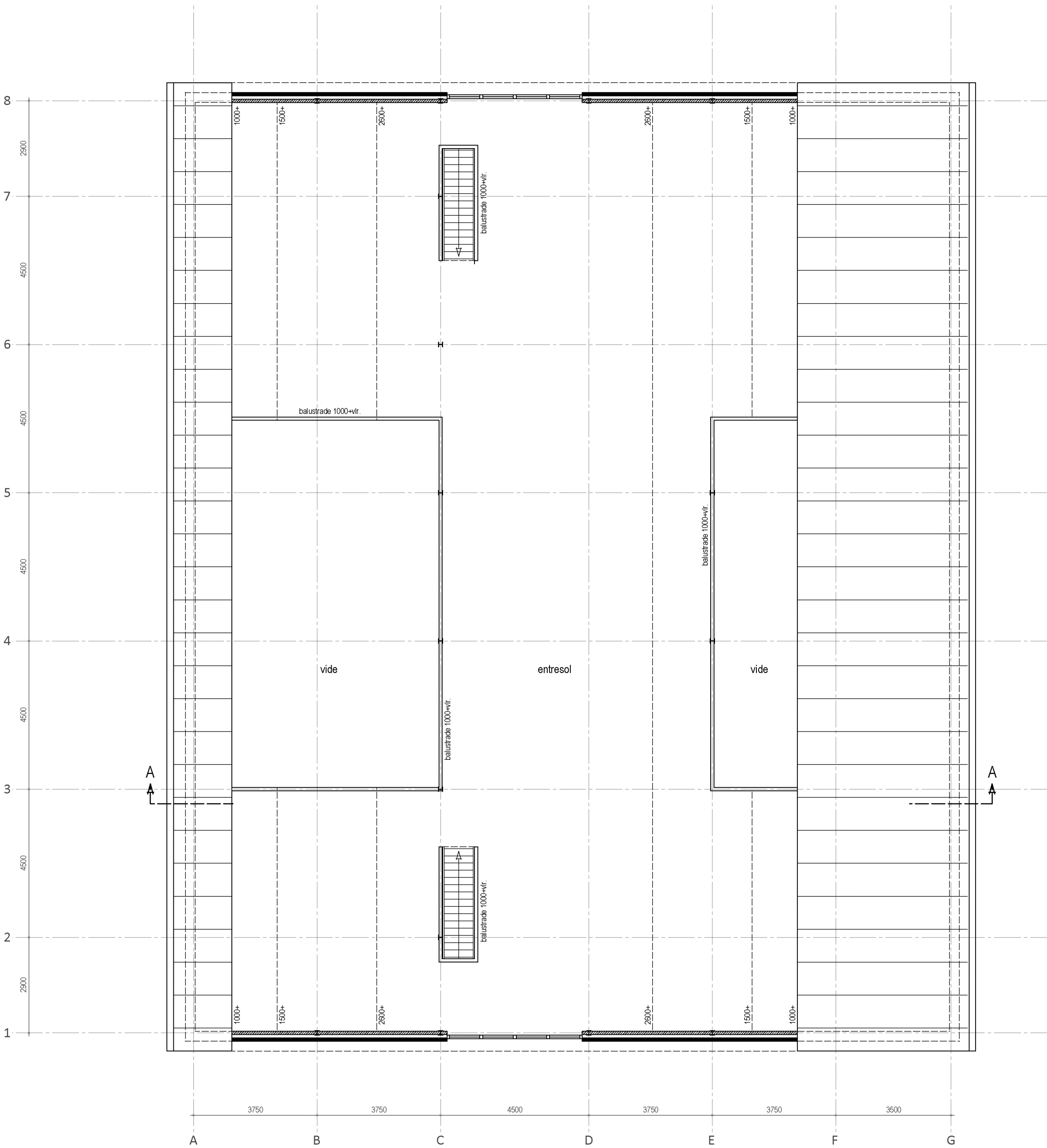
verdieping bestaand
