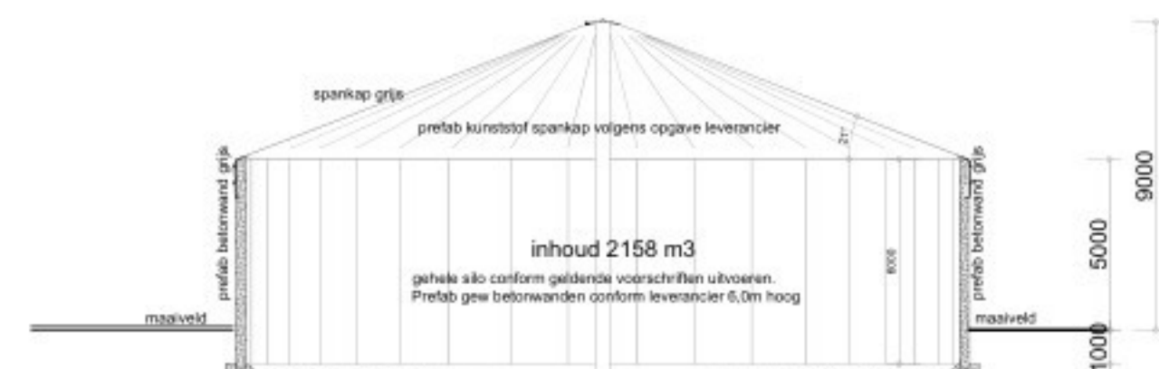
- Doorsnede B - B gebouw 2 -
