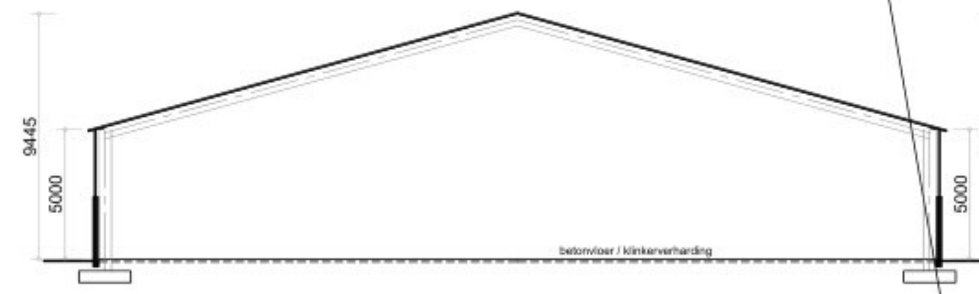
- Doorsnede C - C gebouw 3 -
