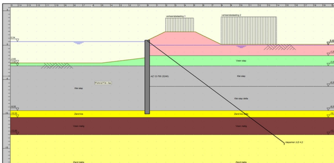
Figuur 2: modellering van de nieuwe damwand volgens de ingediende geotechnische beschrijving
