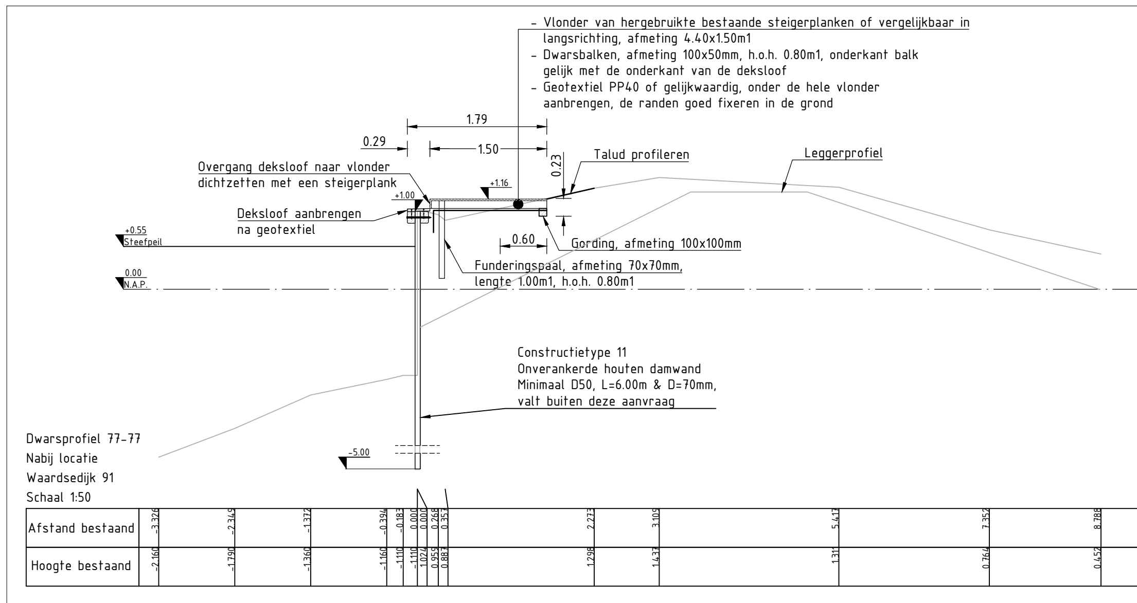
Dwarsprofiel 77-77, schaal 1:50
