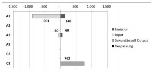
Abb.1: Holzzinzhärente CO 2 -Produktsystemein- und -ausgänge [kg CO 2 -Äqv.]. Die inverse Vorzeichengebung der In- und Outputs trägt der ökobilanziellen CO 2 -Flussbetrachtung aus Sicht der Atmosphäre Rechnung.
