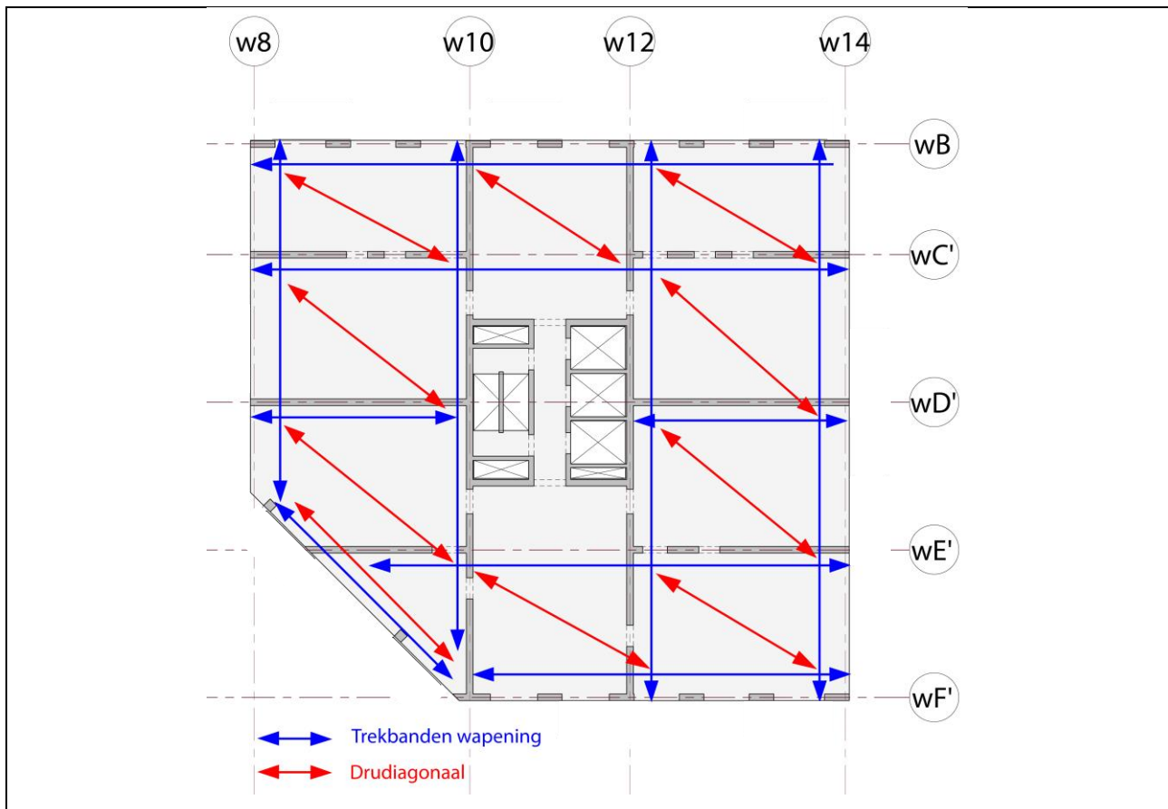
figuur 6: Trekbandwapening voor schijfwerking, tweede draagweg
