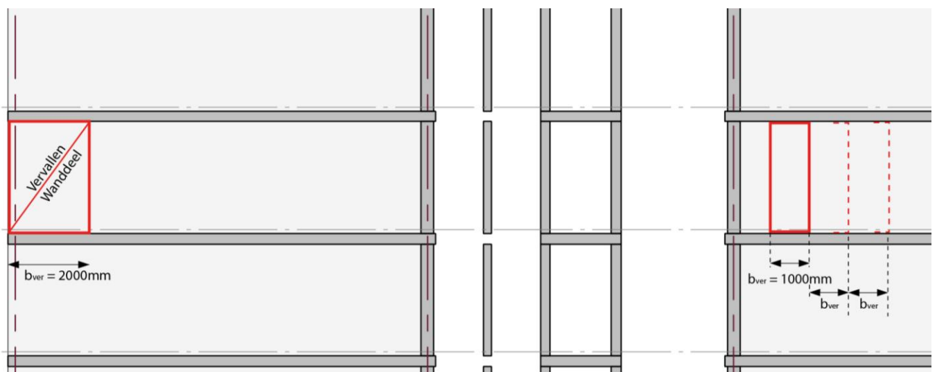
figuur 4: fictief te verwijderen wanddeel in wand wD
