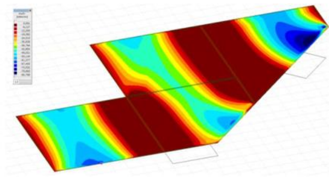
Veldmomenten bij vervallen gevelkolom door calamiteit
