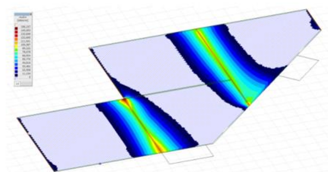
Steunpuntmomenten bij vervallen gevelkolom door calamiteit
