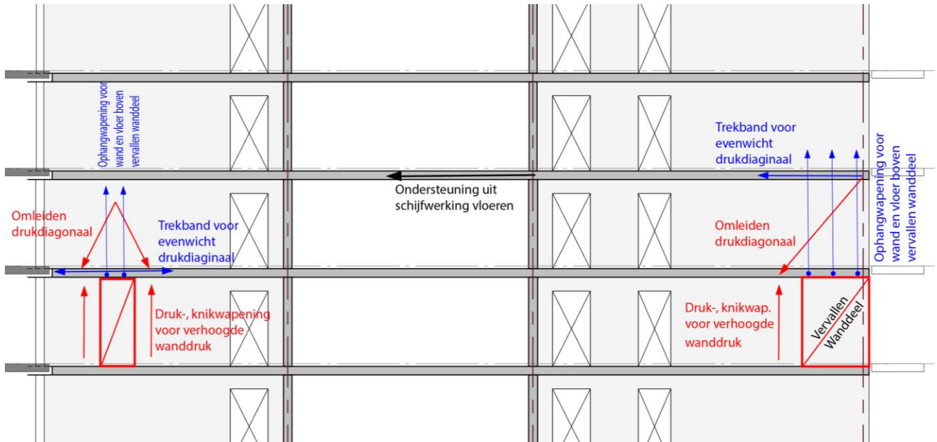
figuur 5 Trekbandvoorzieningen voor tweede draagweg
