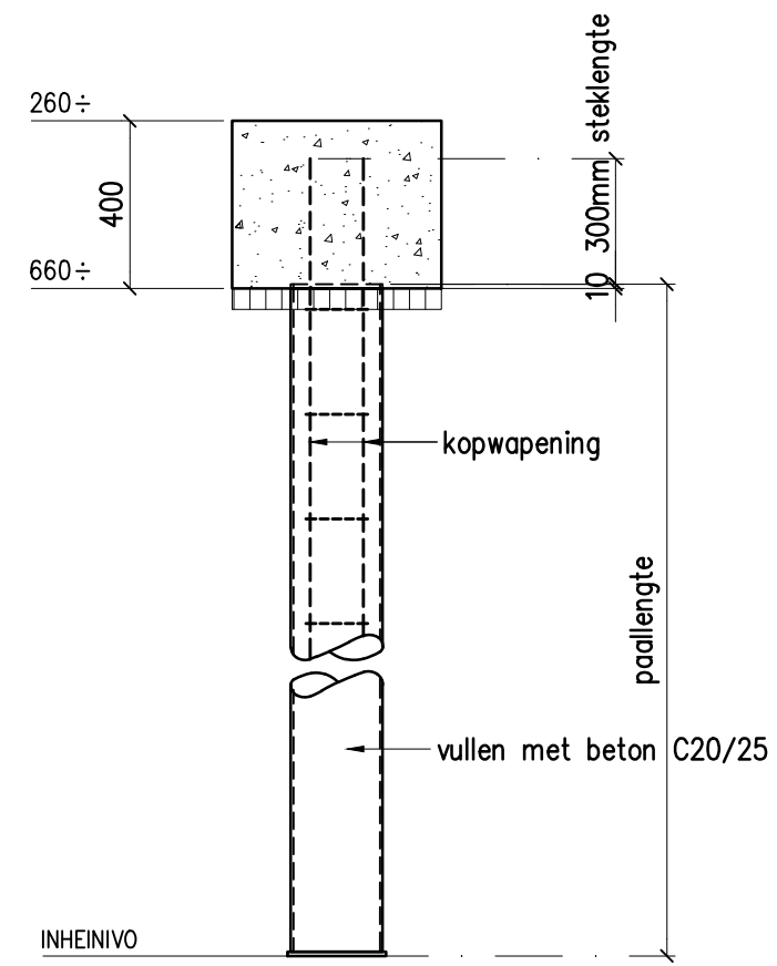
Paaldetail stalen buispaal
