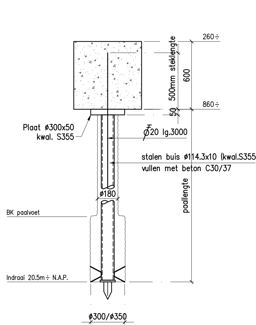
Paaldetail schroefinjectiepaal merk
