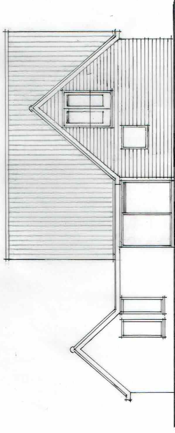
ZUIDGEVEL □ BESTAAND
