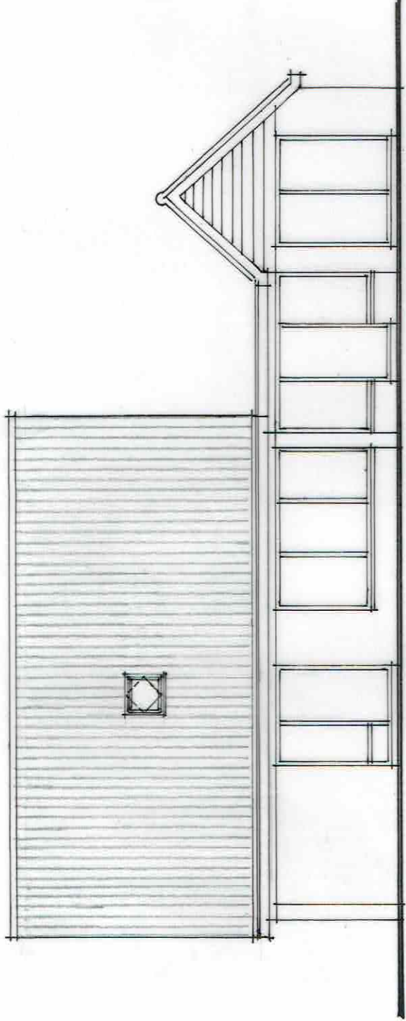
NOORDGEVEL □ BESTAAND
