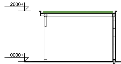
DOORSNEDE
