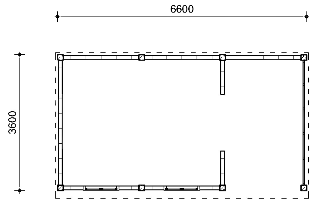
PLATTEGROND
