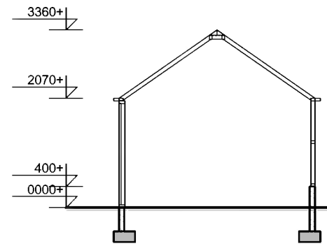
DOORSNEDE
