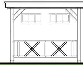
RECHTERZIJGEVEL
