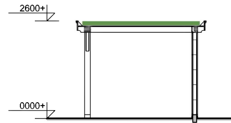
DOORSNEDE
