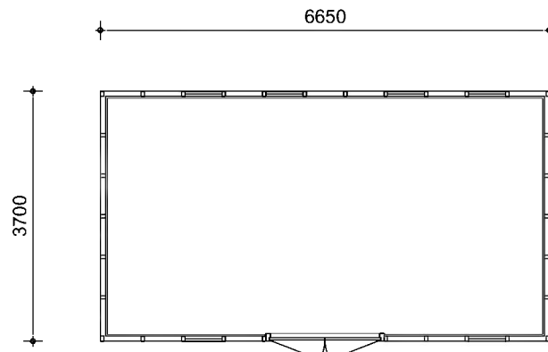
PLATTEGROND
