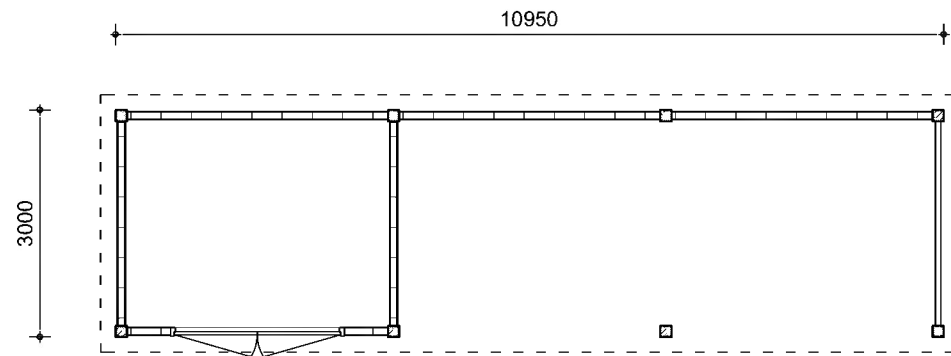
PLATTEGROND
