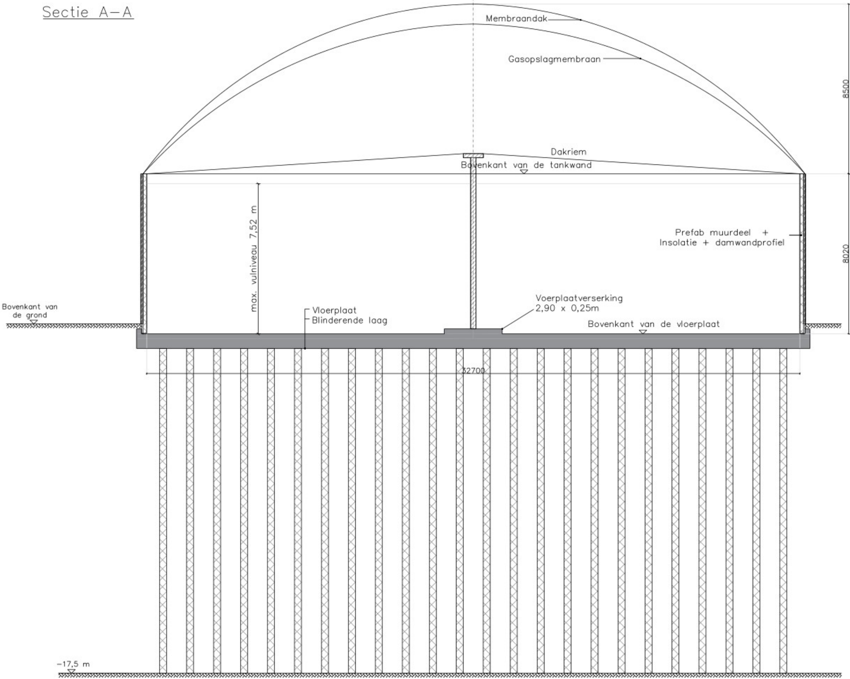
Sectie A-A
