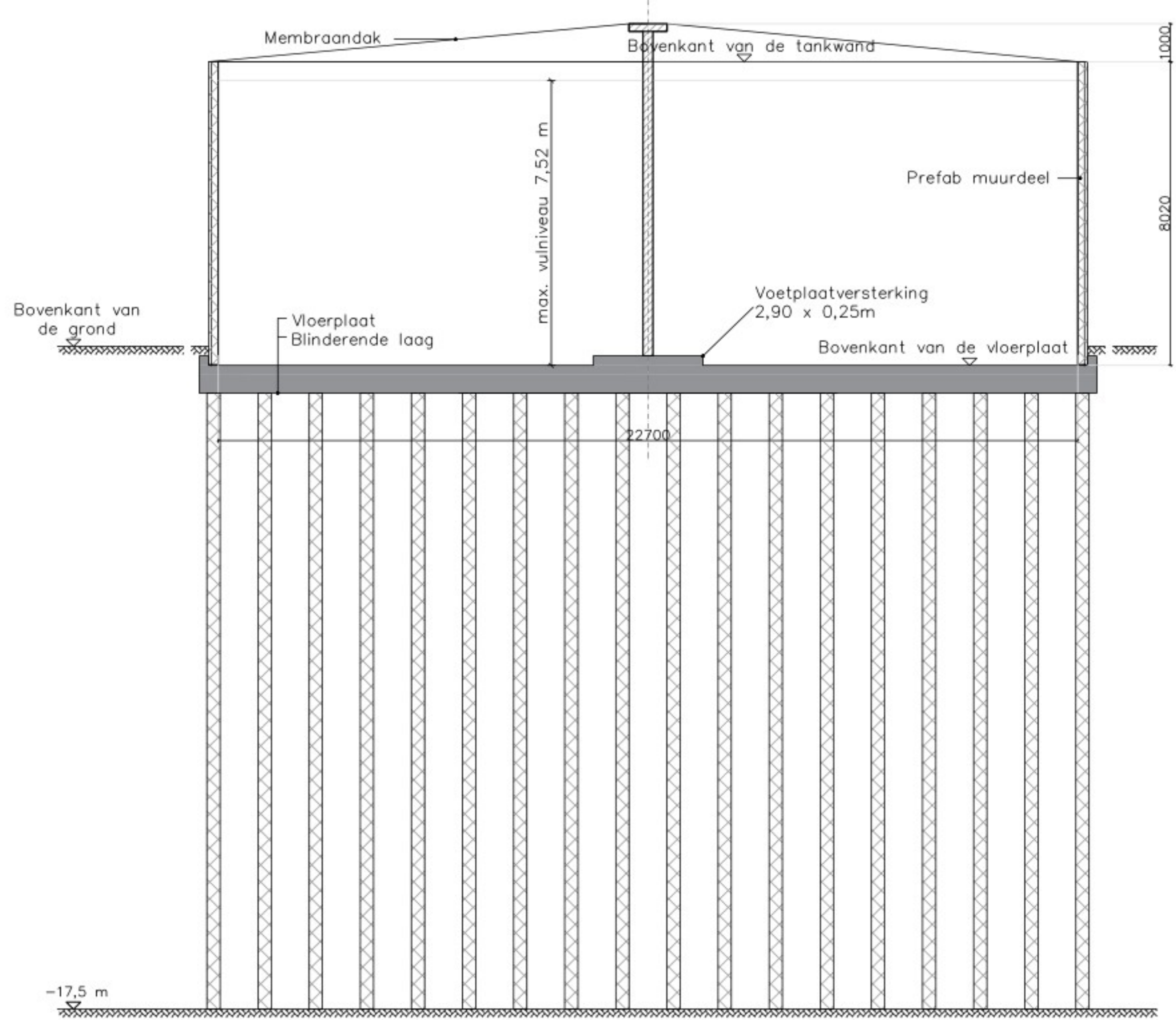
Sectie A-A
