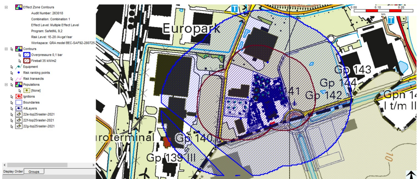
Figuur 8: Explosie-aandachtsgebied
