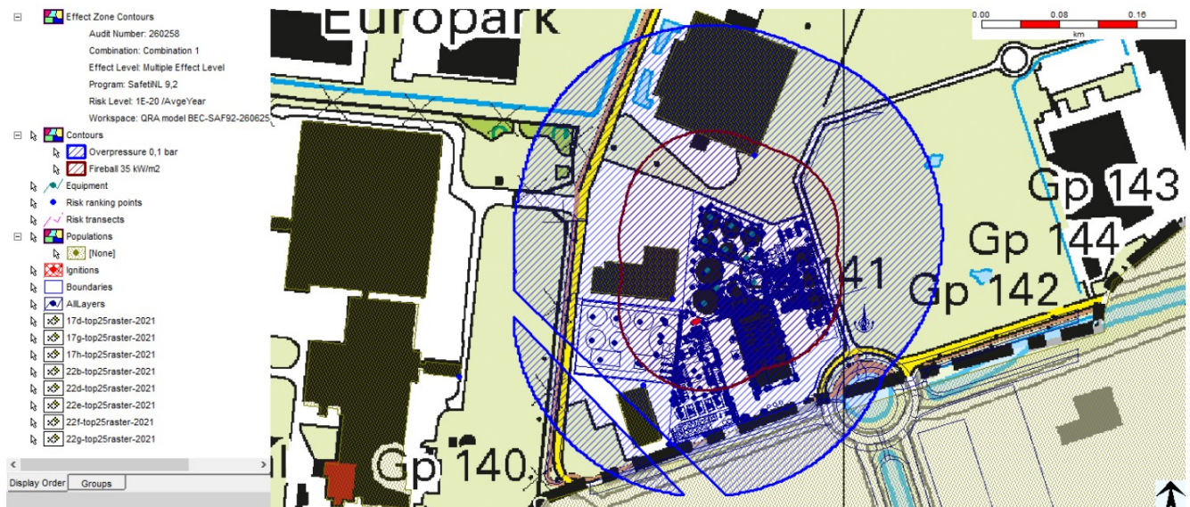
Figuur 7: Explosie-aandachtsgebied
