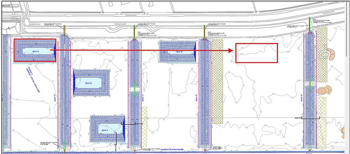
Figuur 1: Situatietekening van de nieuwe locatie van vijver A
