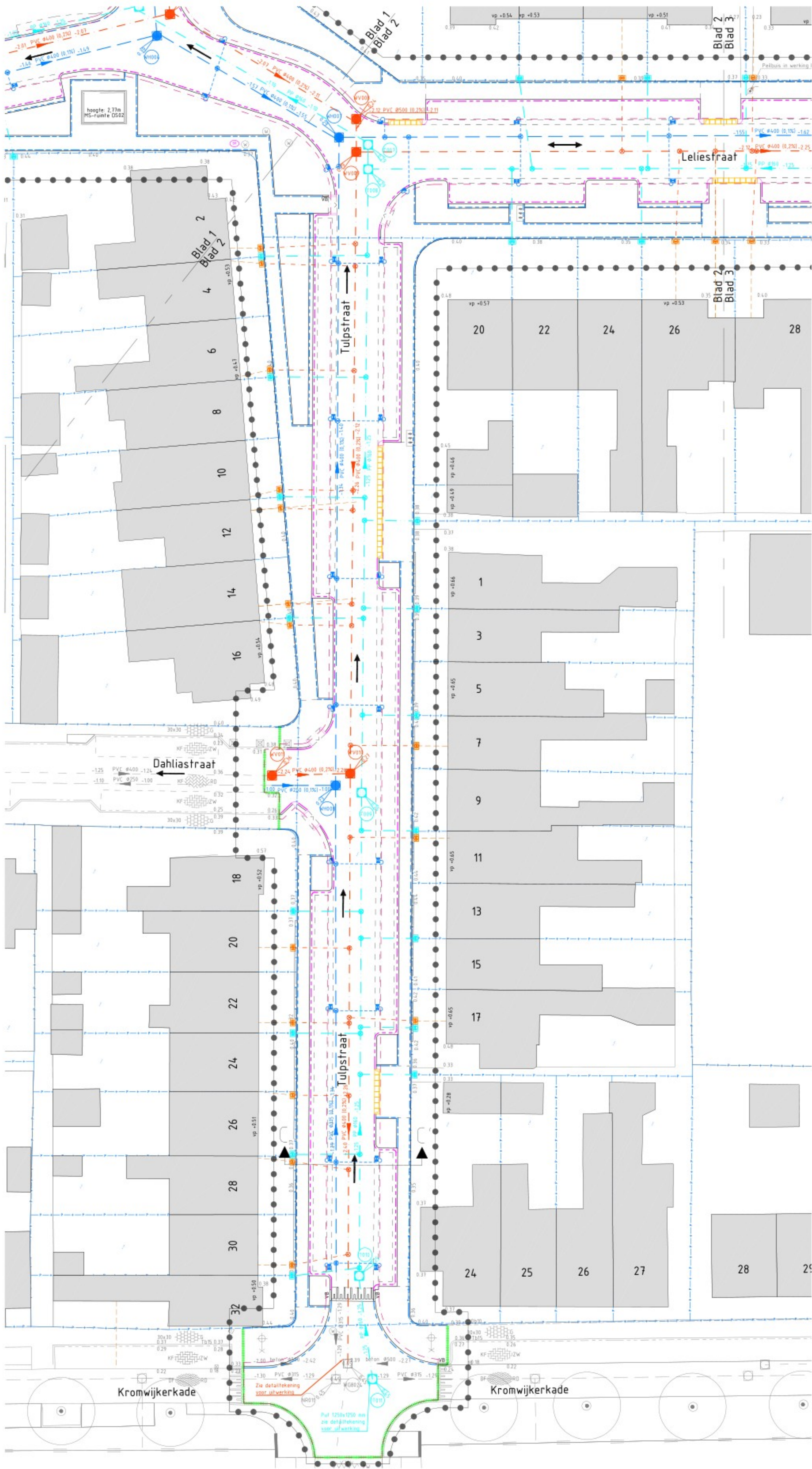
OVERZICHTSTEKENING SCHAAAL 1:200
