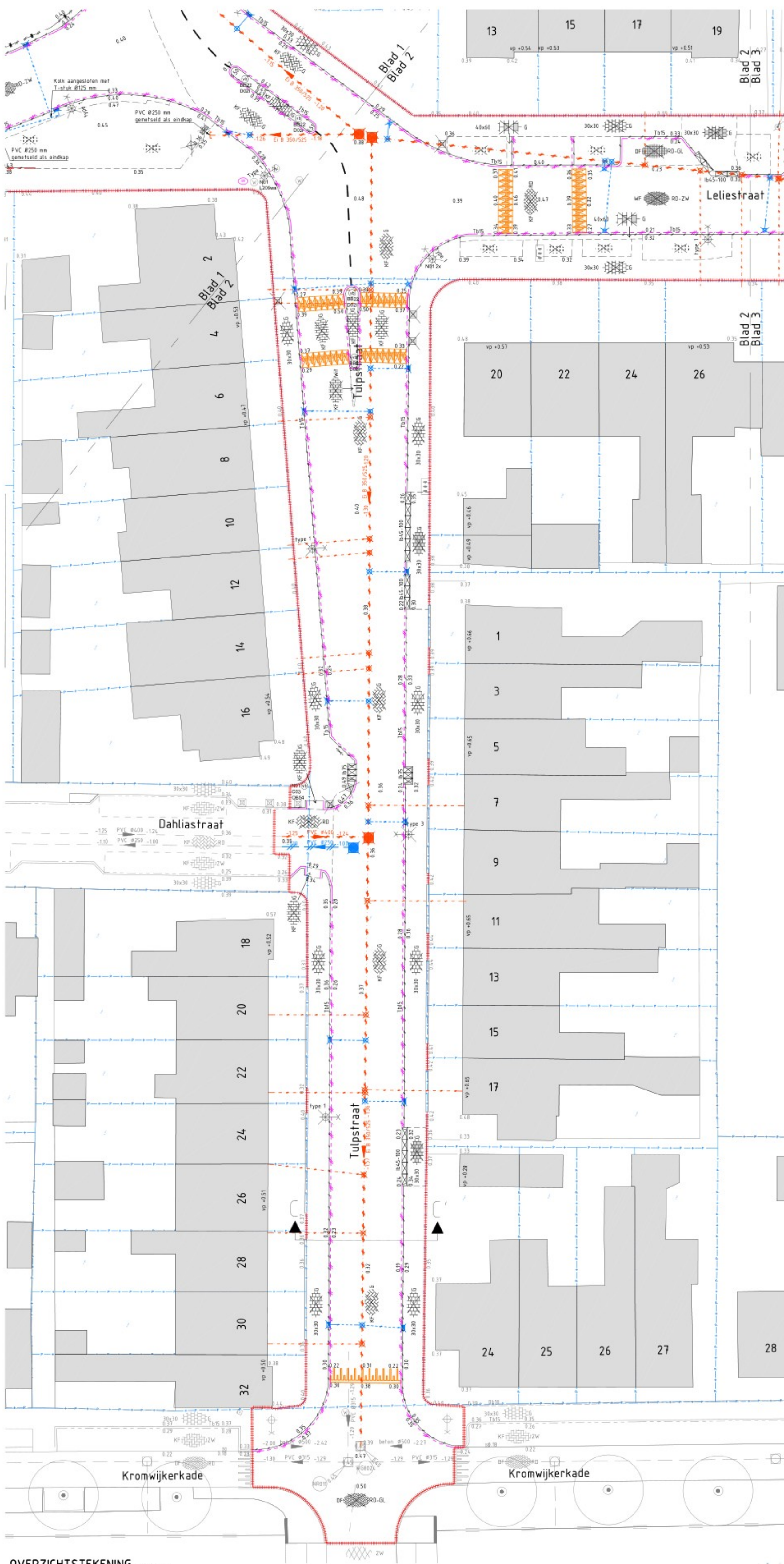
OVERZICHTSTEKENING SCHAAAL 1:200
