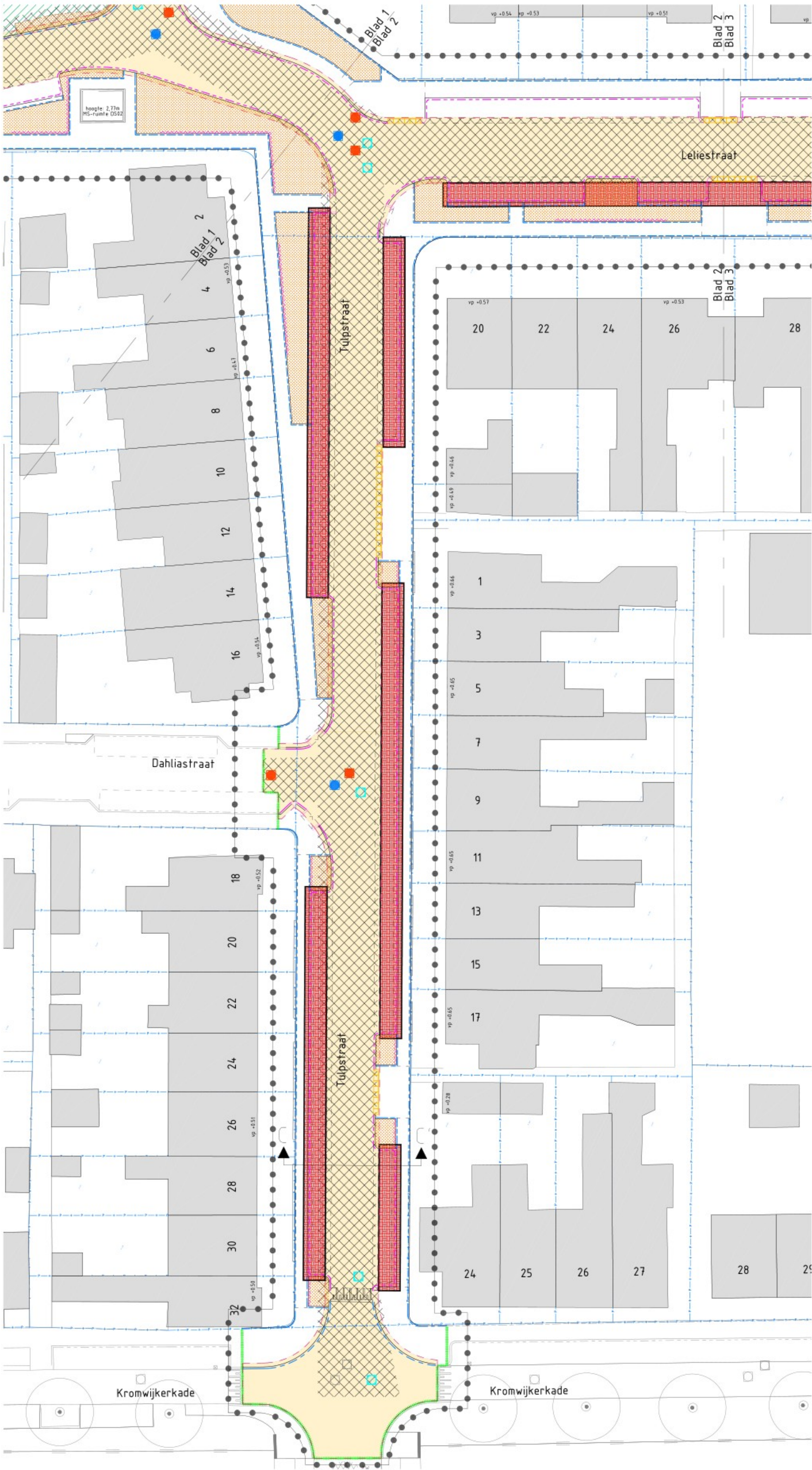
OVERZICHTSTEKENING SCHAAAL 1:200
