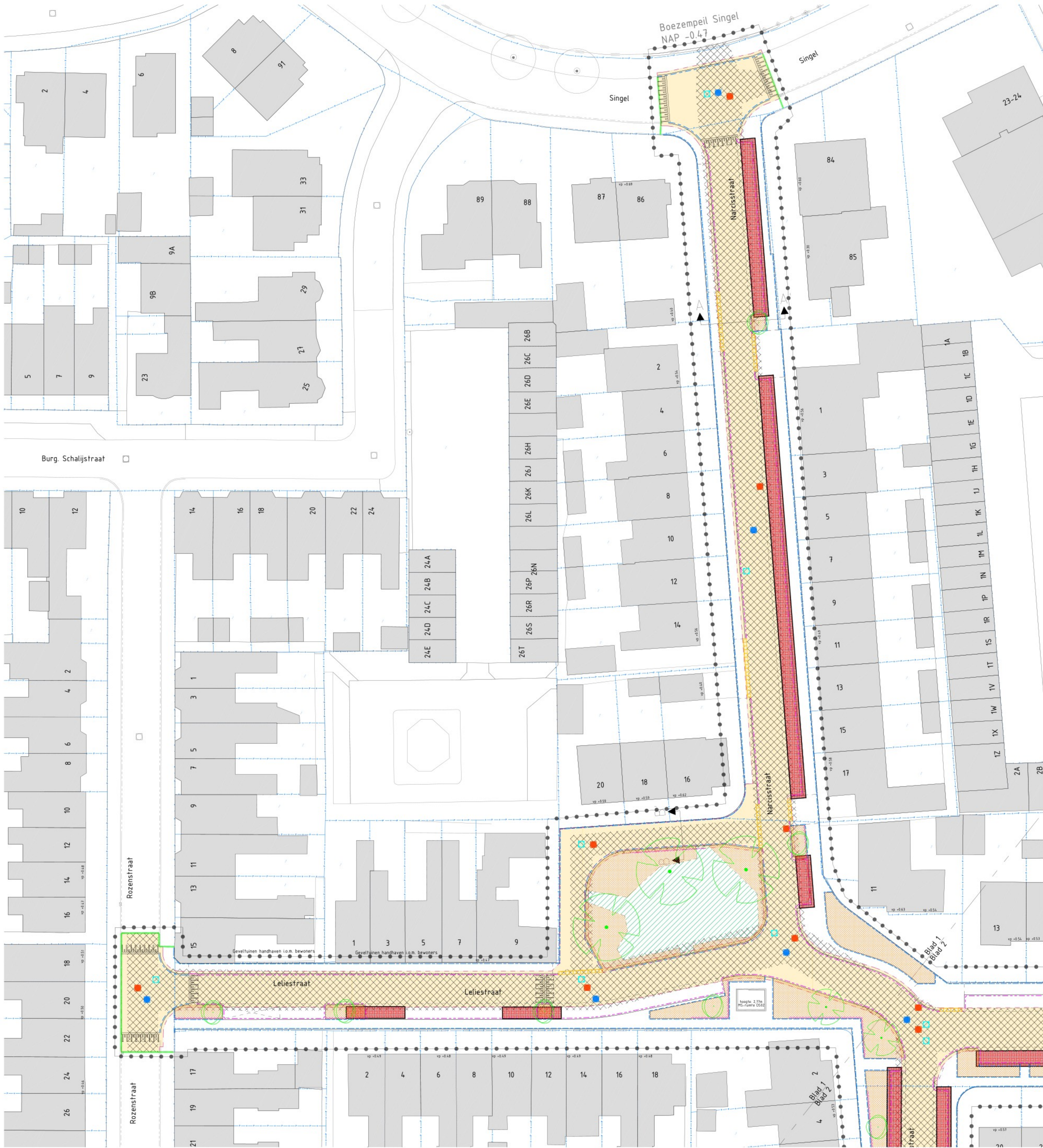
OVERZICHTSTEKENING SCHAAF 1:200
