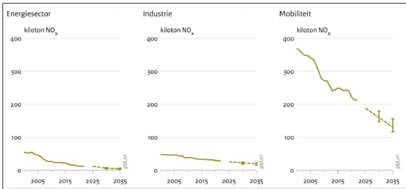
Afbeelding 3 Ontwikkeling van de NOx-emissie van de sectoren energie, industrie en mobiliteit. Bron: Zie voetnoot 6
