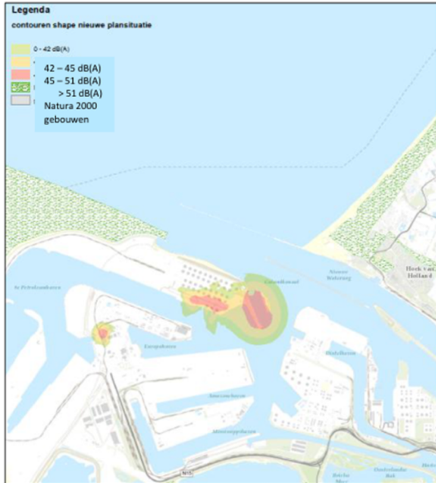
Figuur 5-1: Geluidbelasting vanuit Gate terminal
