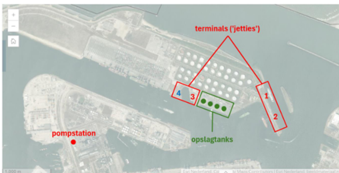
Afbeelding 3.1 Ligging van Gate Terminal met Jetty 1 - 4
