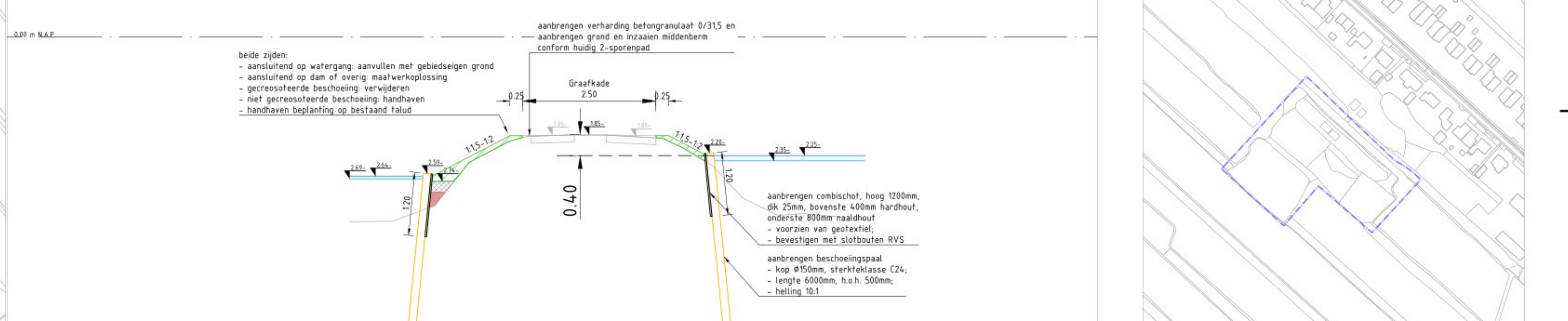
Dwarsprofiel GK 6-6' SCHAAL 1 : 50
