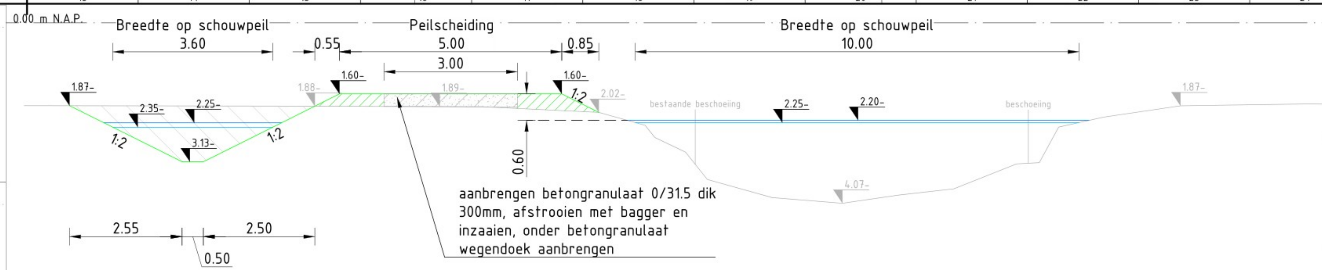
Dwarsprofiel GK 9-9' SCHAAL 1 : 50
