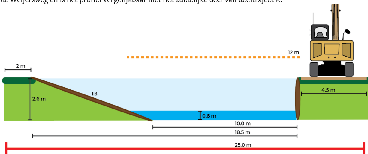
Figuur 4-6: Principe profiel deeltraject A, inpassing terrein voormalige dakpannenfabriek
