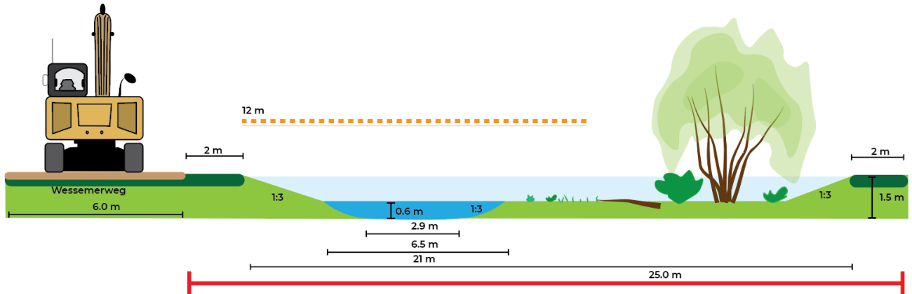
Figuur 4-13: Principe profiel deeltraject C ten oosten van de Oellestraat met onderhoud vanaf de Wessemerweg.
