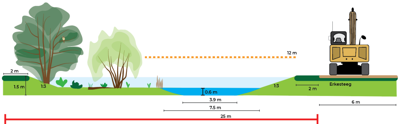
Figuur 4-8: Principe profiel deeltraject B ten westen van de voorde.
