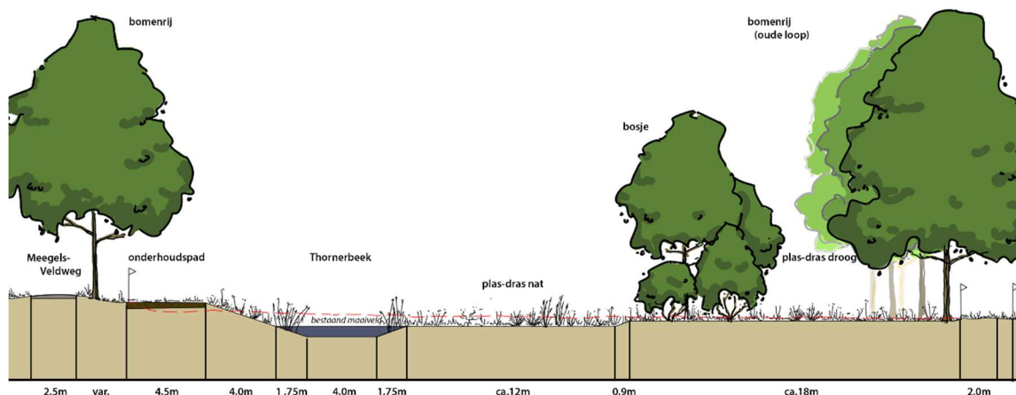
Figuur 5-26 Doorsnede t.h.v. laagte met naast de watergang een zeer licht oplopend talud met een natte en iets drogere zone.
