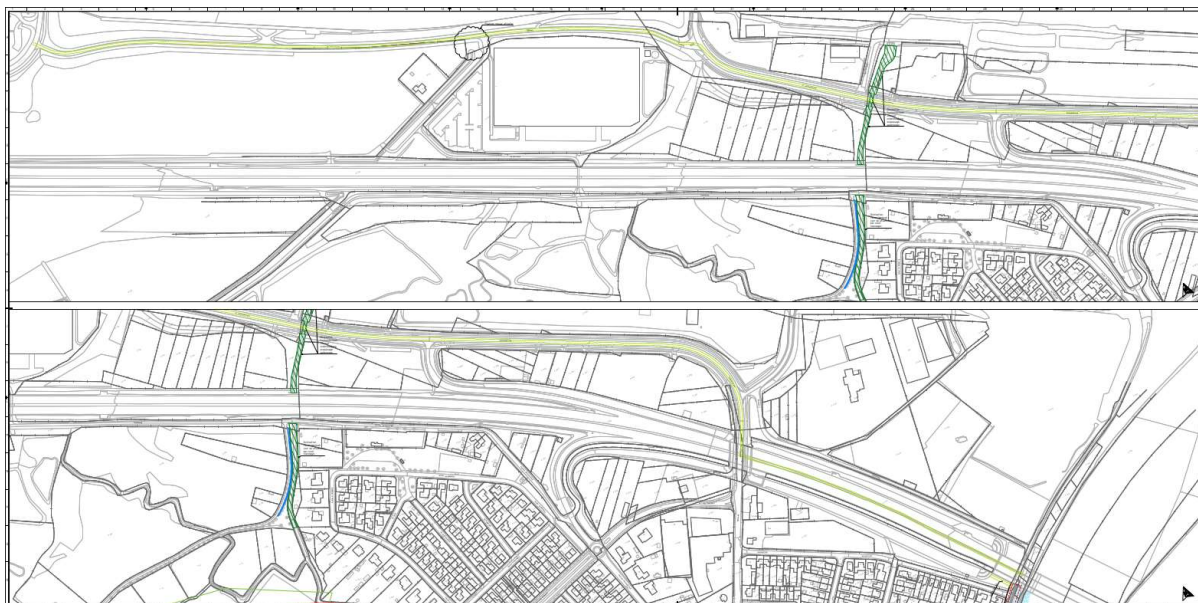
Figuur 4-32 Ontwerptekening verholten kering (dijksectie 5)
