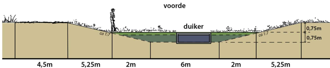
Figuur 5-10 Principedoorsnede doorwaadbare plaats: voorde met duiker
