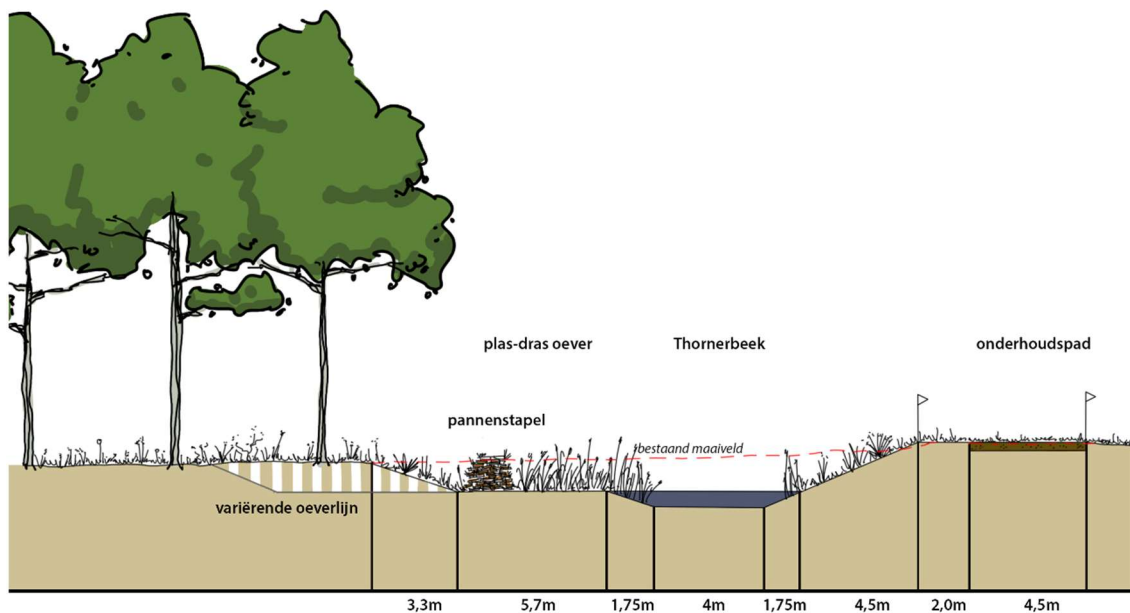
Figuur 5-15 Doorsnede t.h.v. Erkesteeg
