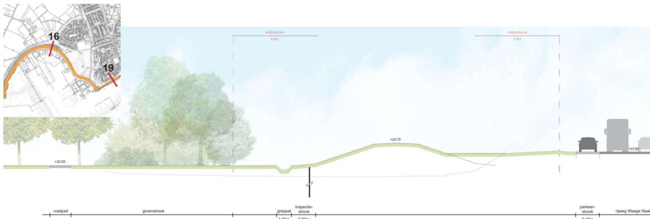
Figuur 4-14 Doorsnede 16 nabij de verbindingsweg naar de Waage Naak
