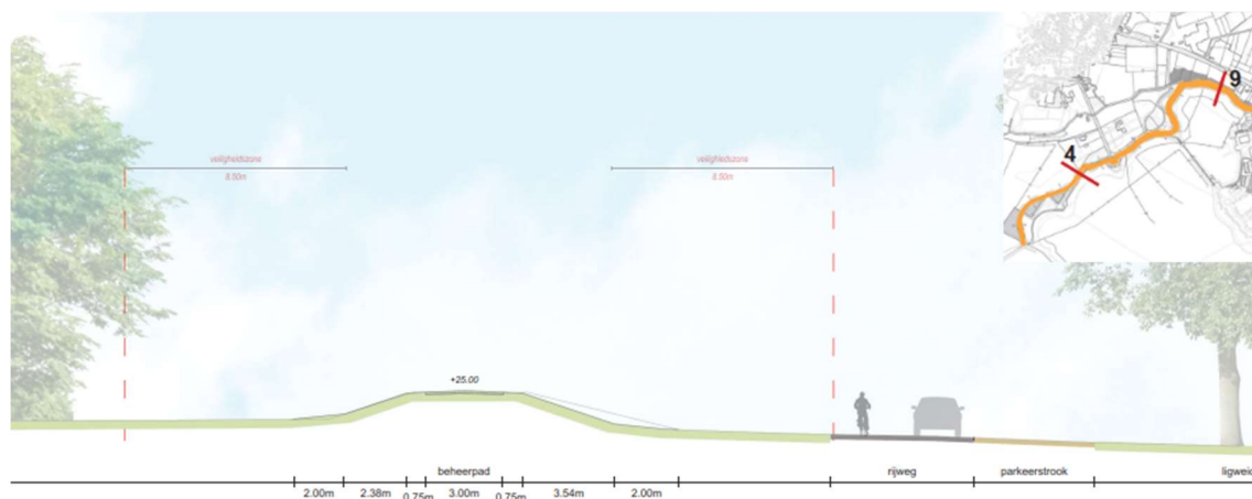
Figuur 4-4 Doorsnede 4 ter plaatse van dagstrandrecreatie
