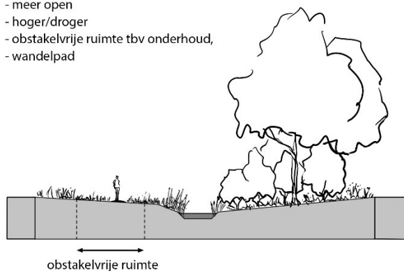
Figuur 5-3 Landschappelijke inpassing principeprofiel R-type 5 voor de Thornerbeek
