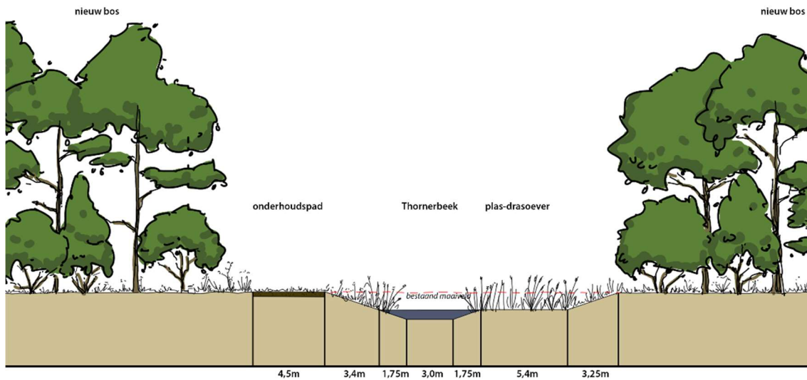
Figuur 5-19 Doorsnede t.h.v. Meggerveld
