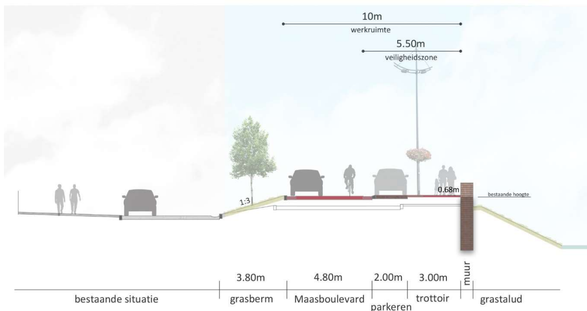
Figuur 4-20 Doorsnede over de Beekstraat en de Maasboulevard, een verhoogd maaiveld vergroot de beleving van het water
