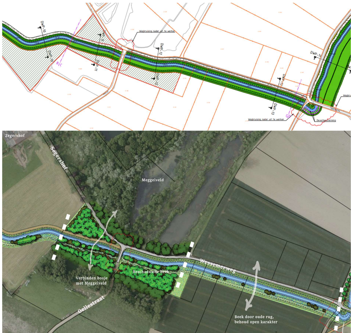
Figuur 5-16 Deeltraject C. Boven: inpassend ontwerp. Onder: Luchtfoto met landschappelijke inpassing.
