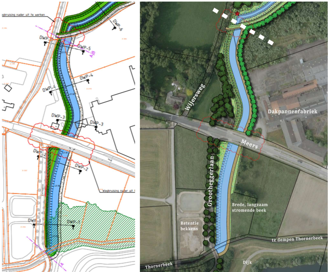
Figuur 5-4 Deeltraject A. Links: inpassend ontwerp. Rechts: Luchtfoto met landschappelijke inpassing.
