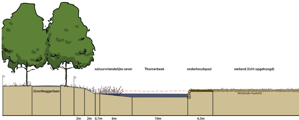
Figuur 5-5 Doorsnede t.h.v. Grootheggerlaan
