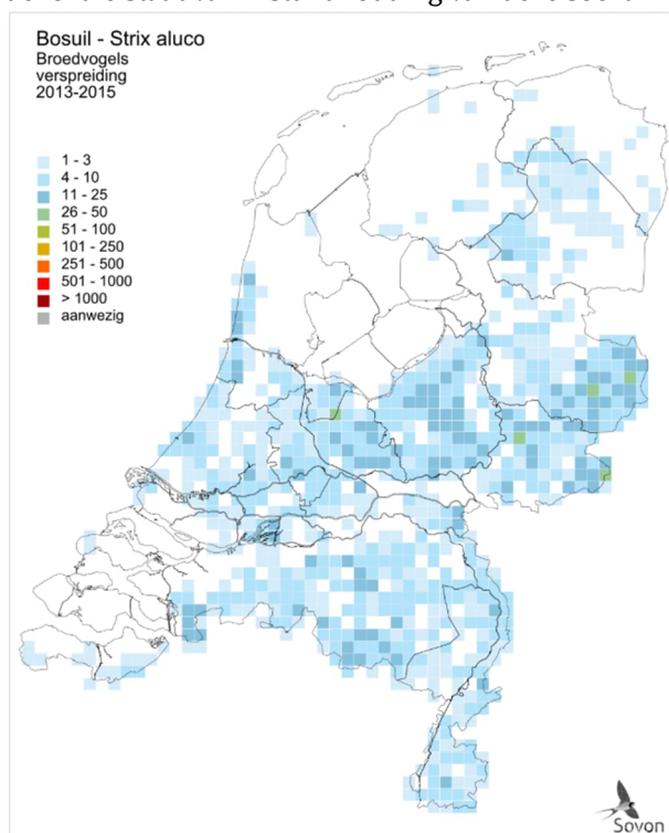
Afbeelding 8-1: verspreiding van de bosuil (Sovon, 2025).
